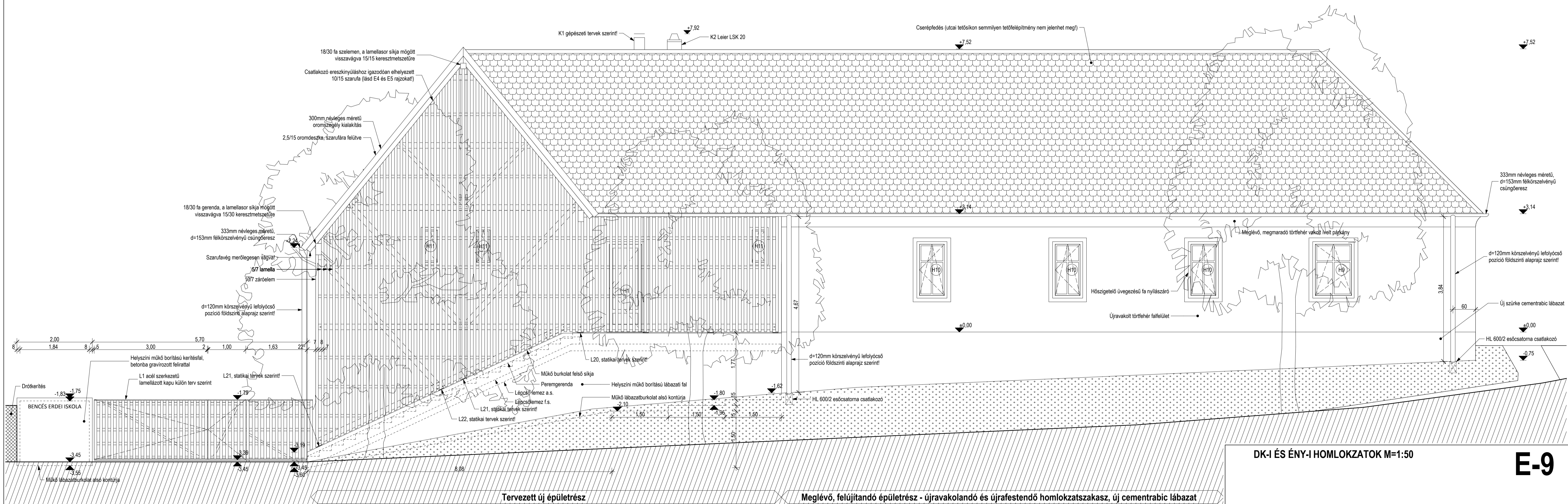
ÉSZAK-NYUGATI HOMLOKZAT M=1:50
