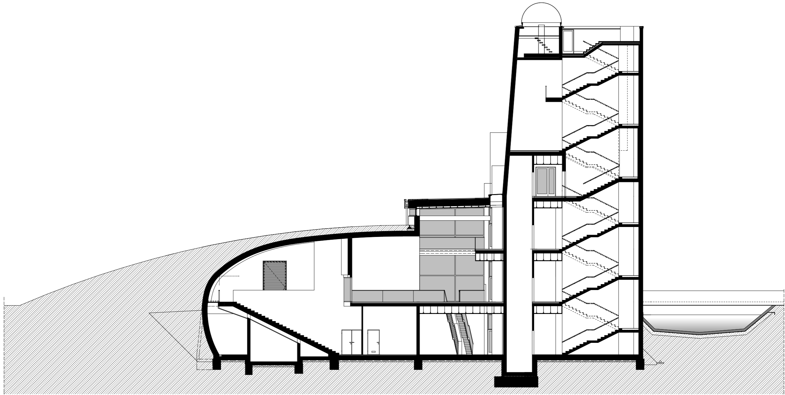
L-L METSZET
