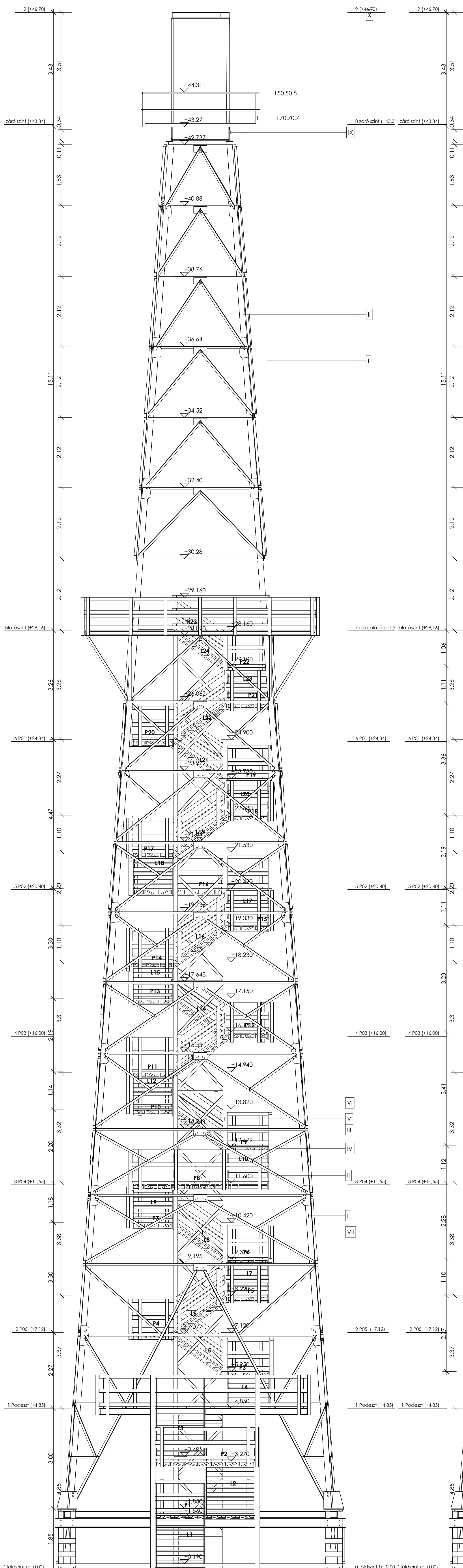
DÉLI HOMLOKZAT m1:50
