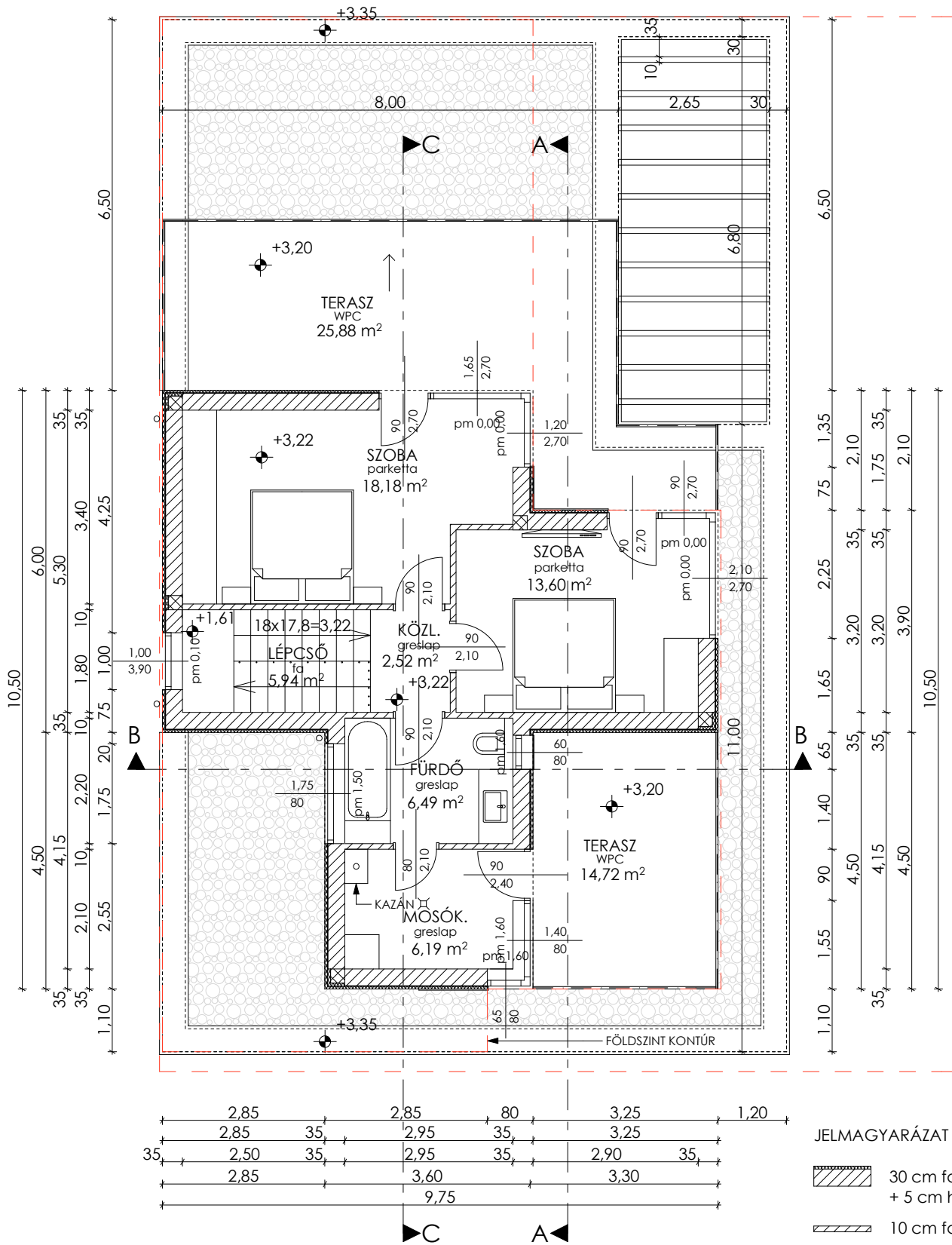
EMELETI ALAPRAJZ
