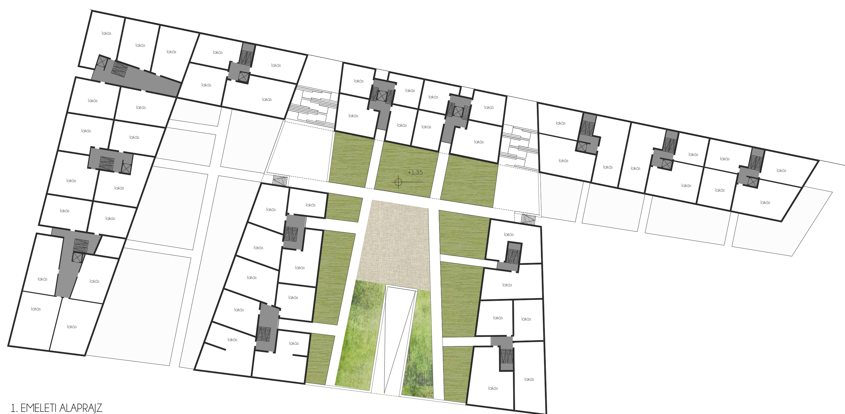
1. EMELETI ALAPRAJZ
