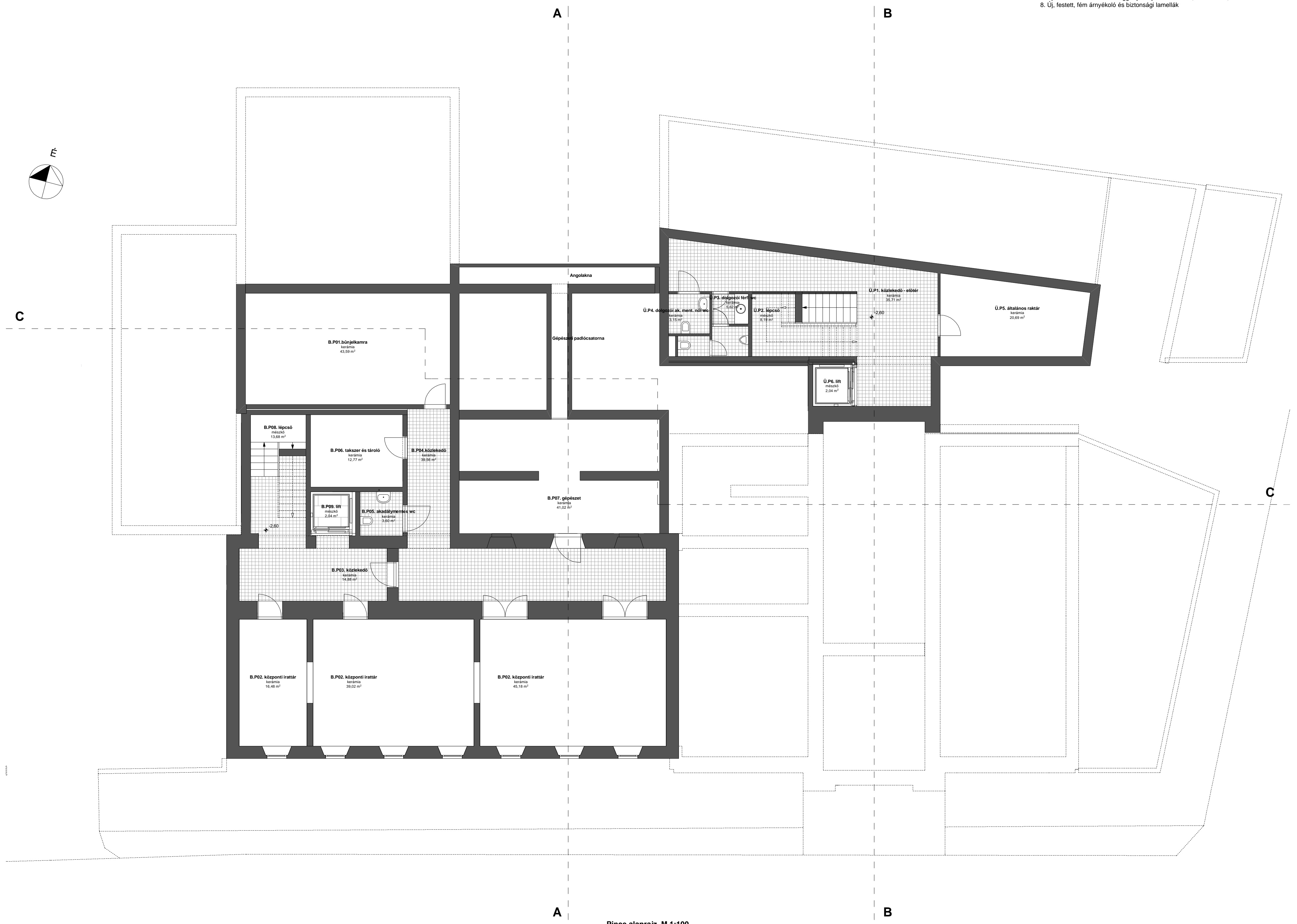
Pince alaprajz M 1:100
