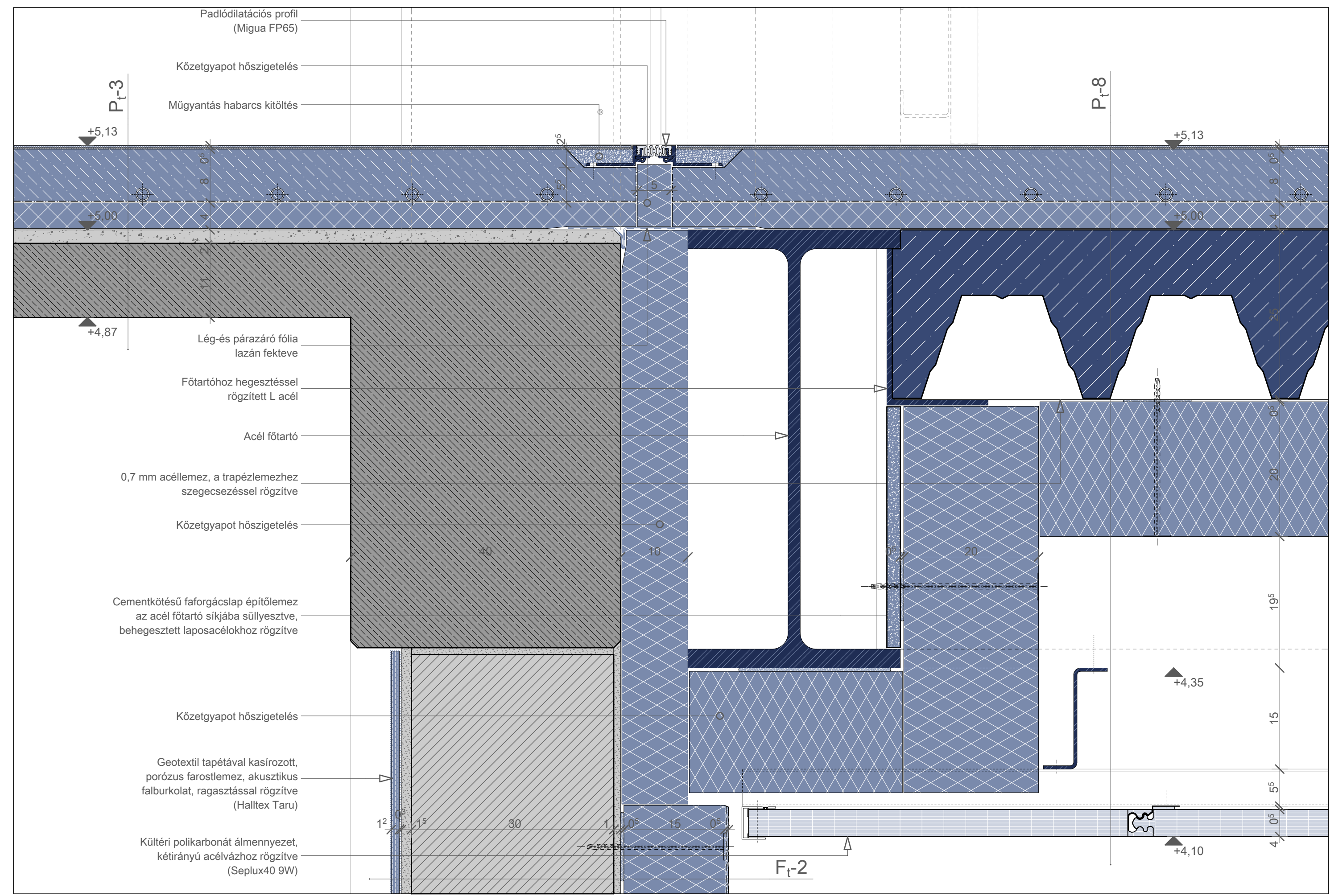
Meglévő- és új épület csatlakozása (alaprajzi részlet)
