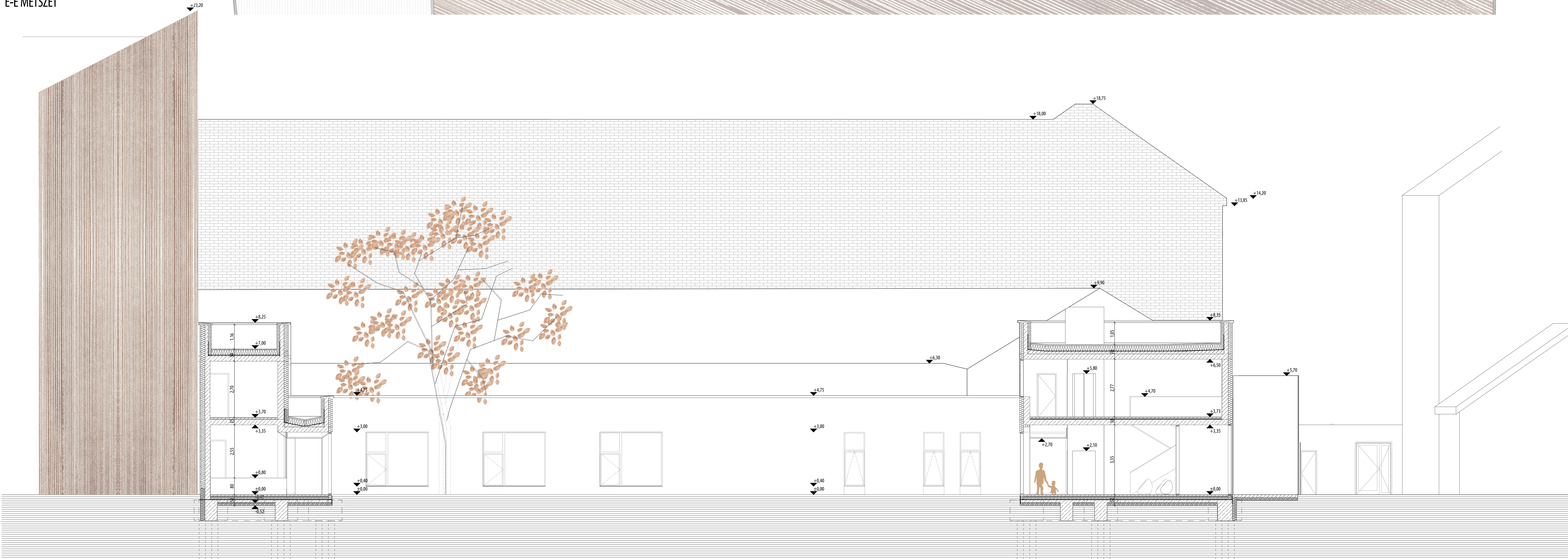
E-E METSZET
