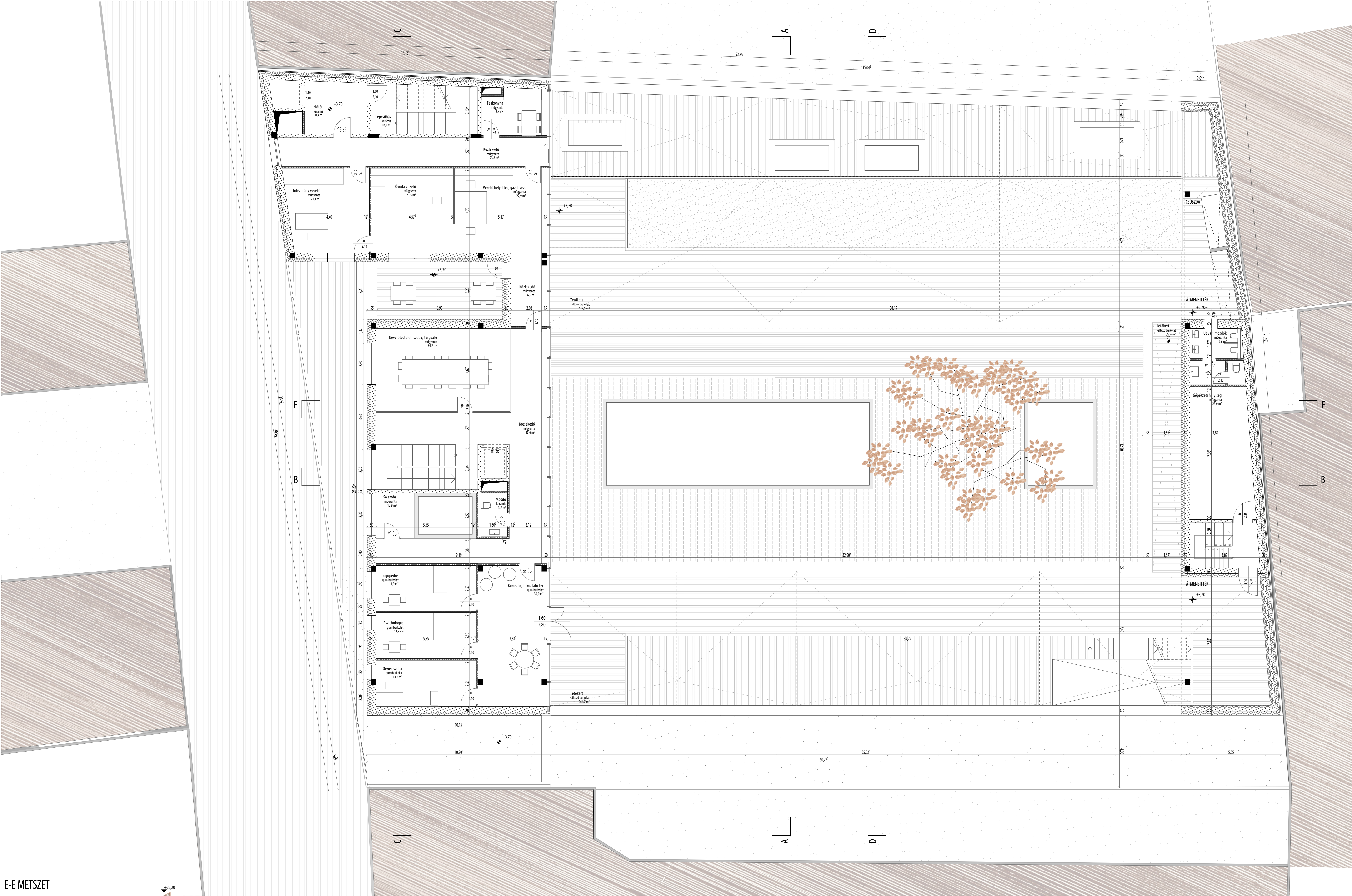
E-E METSZET
