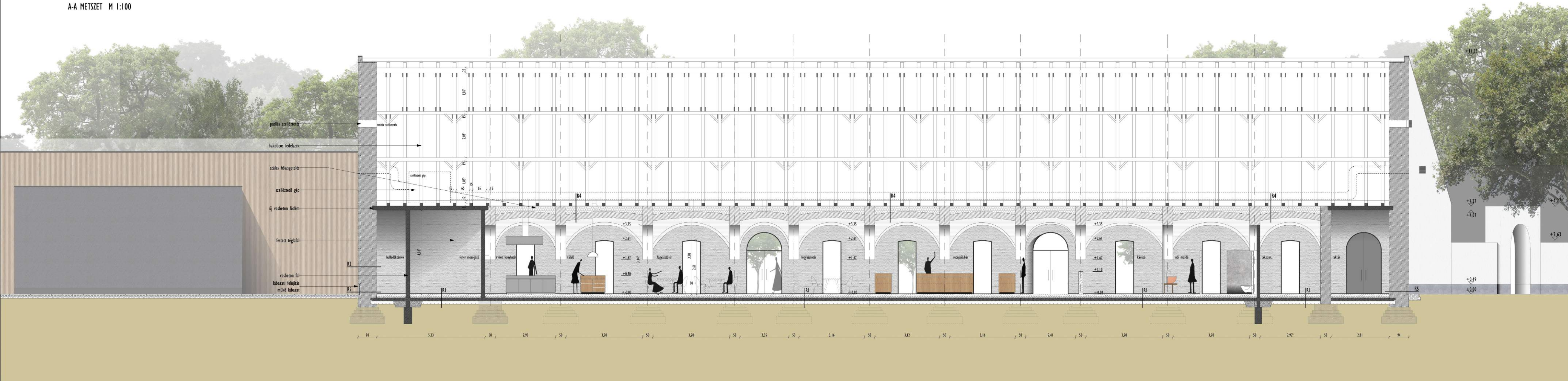
A-A METSZET M 1:100
