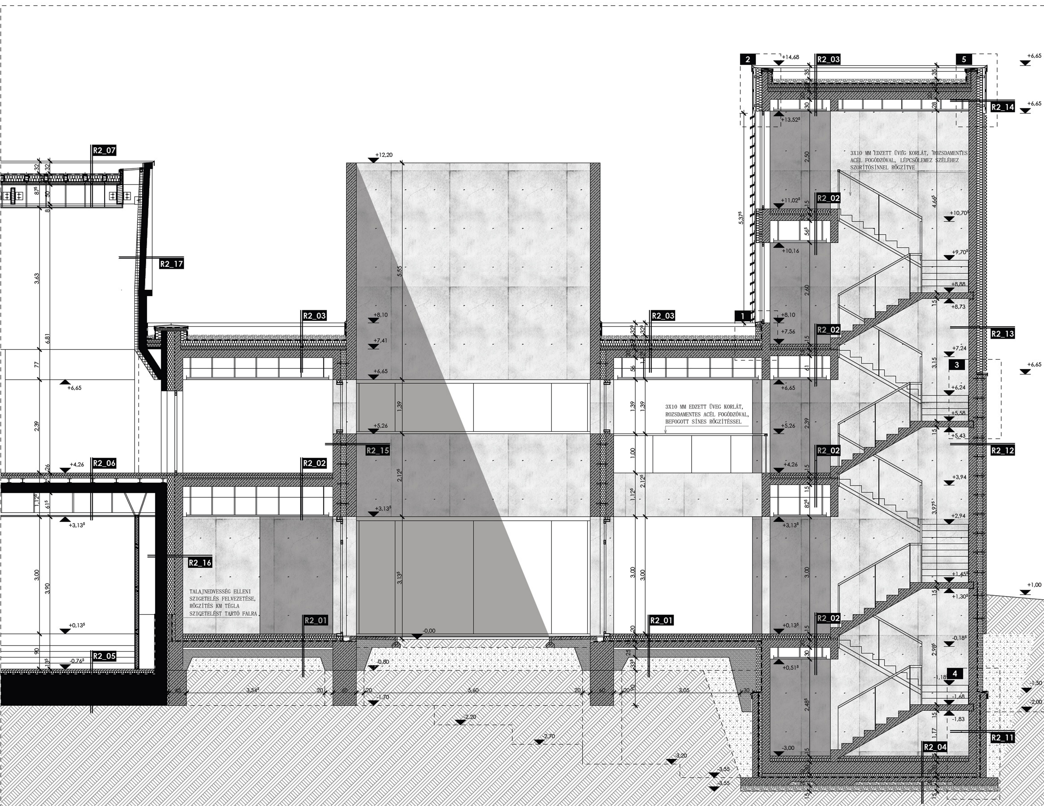
1-1 METSZET M= 1:50
