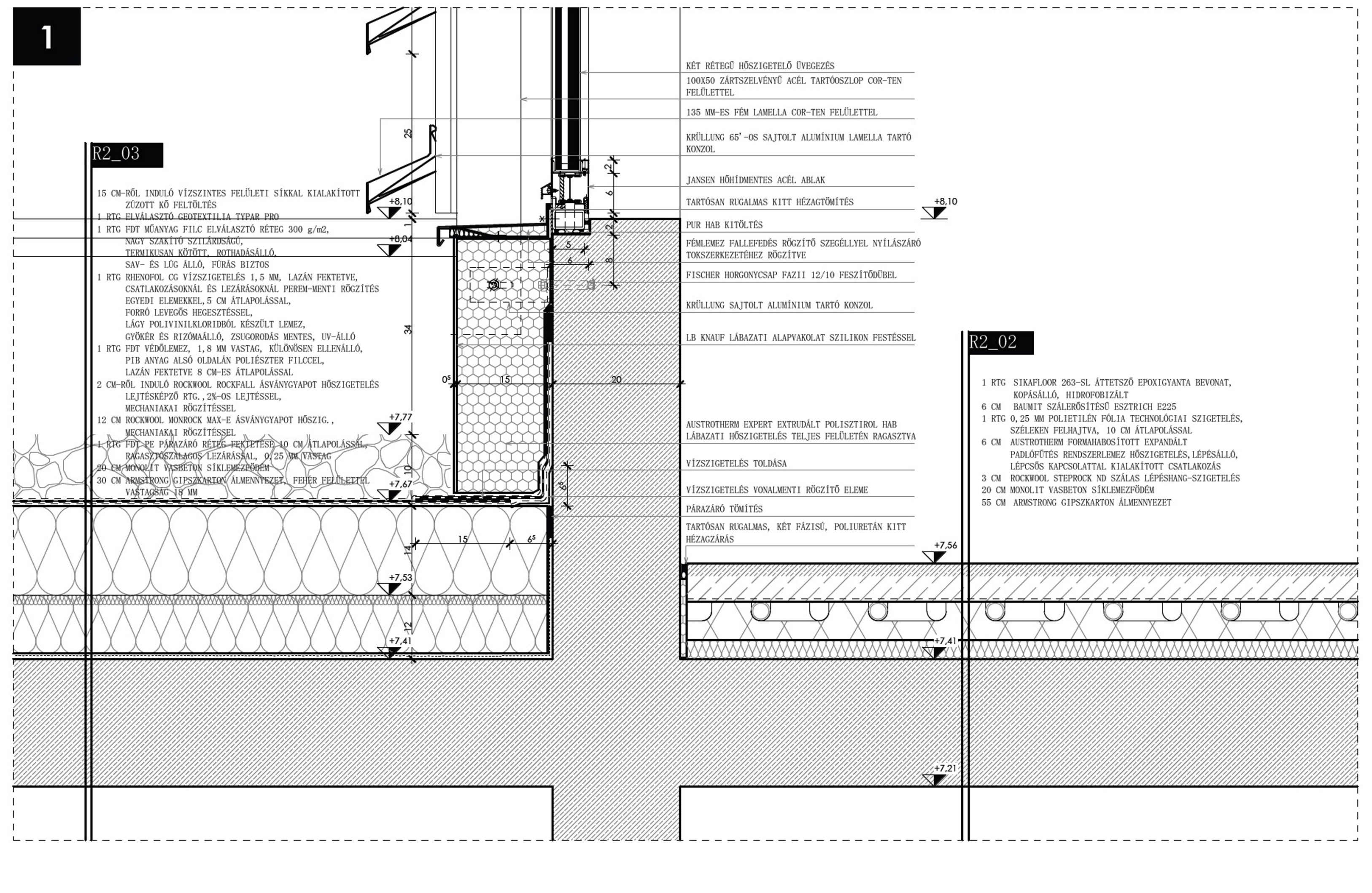
METSZET M=1:50
