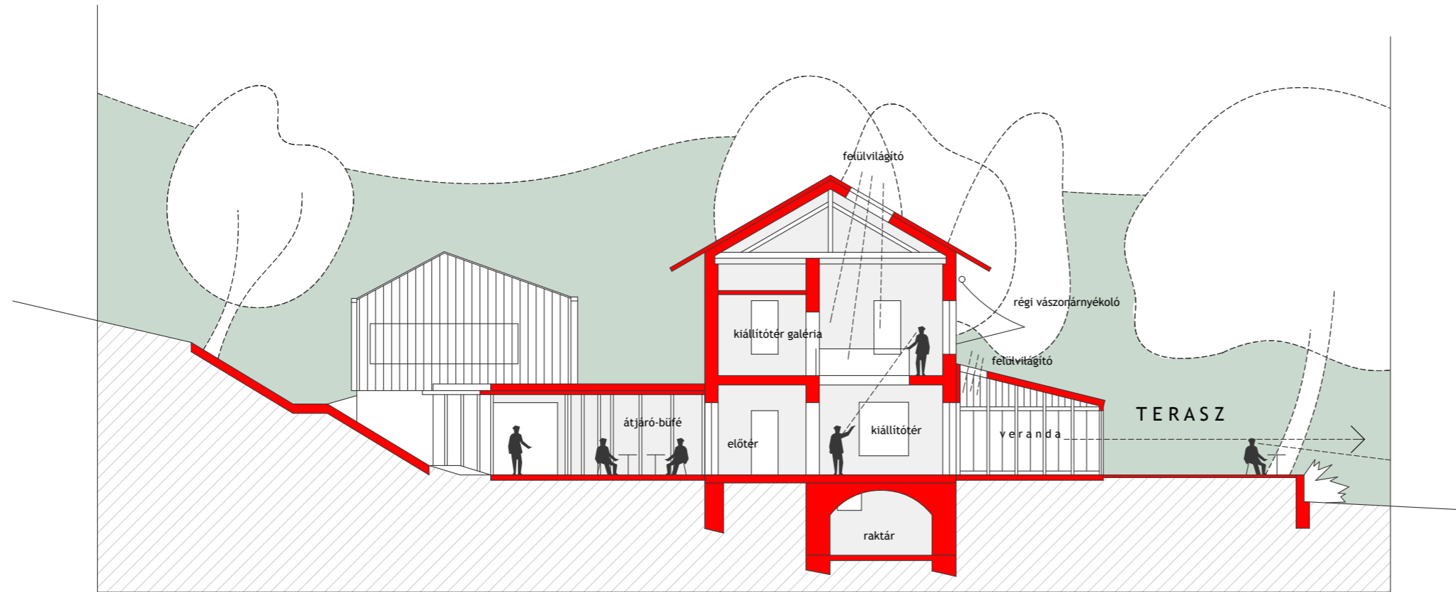
D-D METSZET
