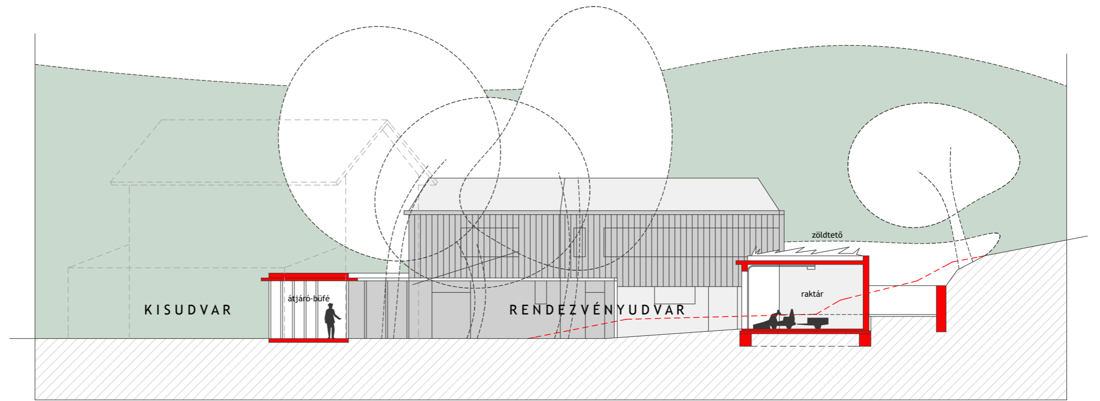
C-C METSZET
