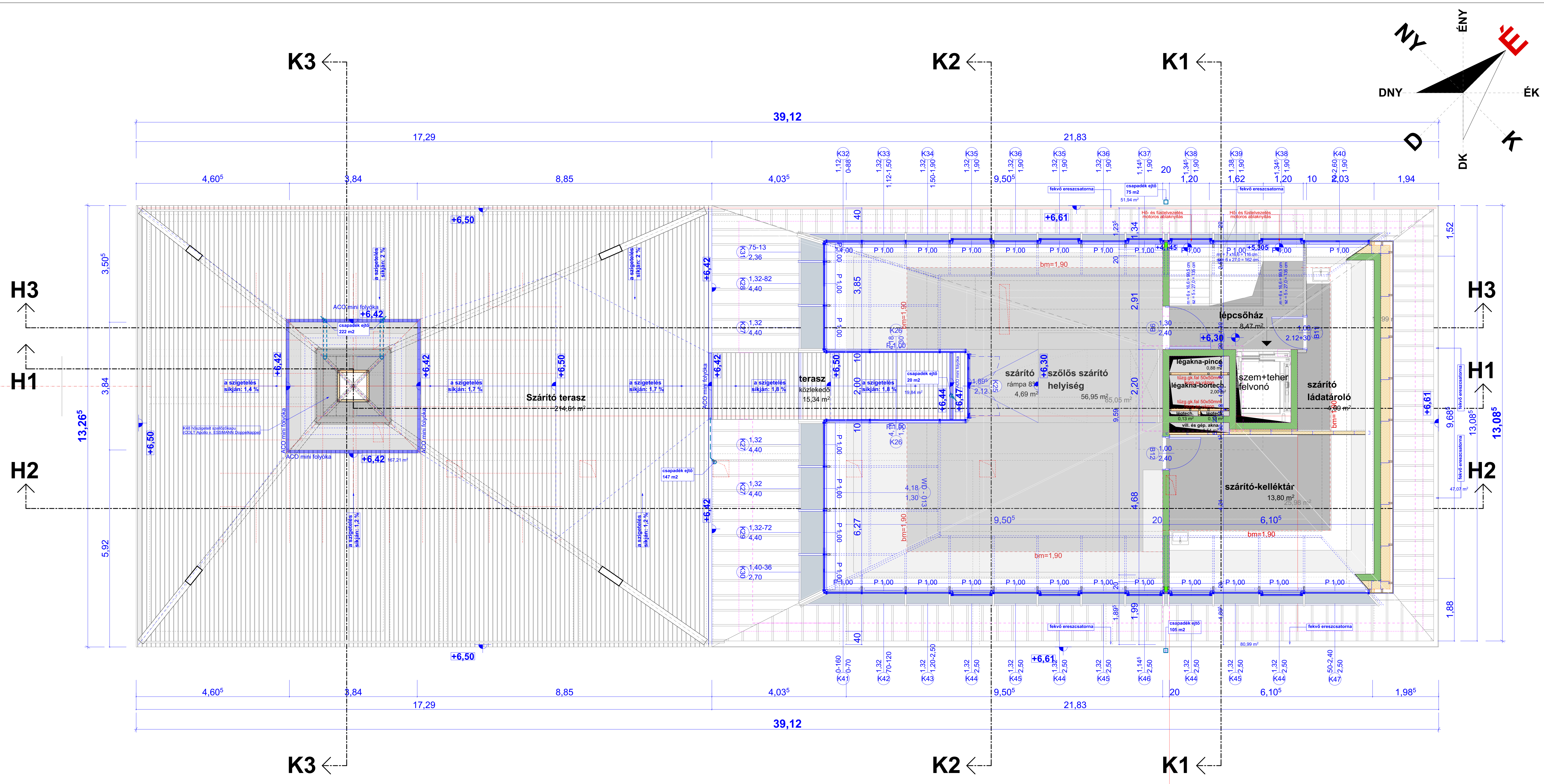
Tetőszinti alaprajz
