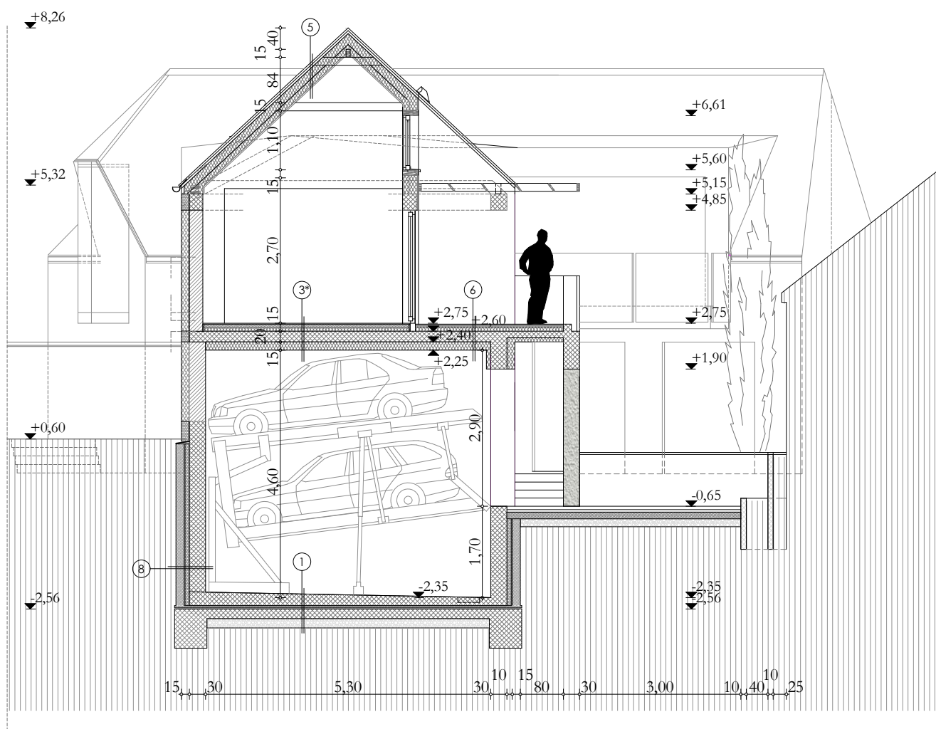
2-2 METSZET
