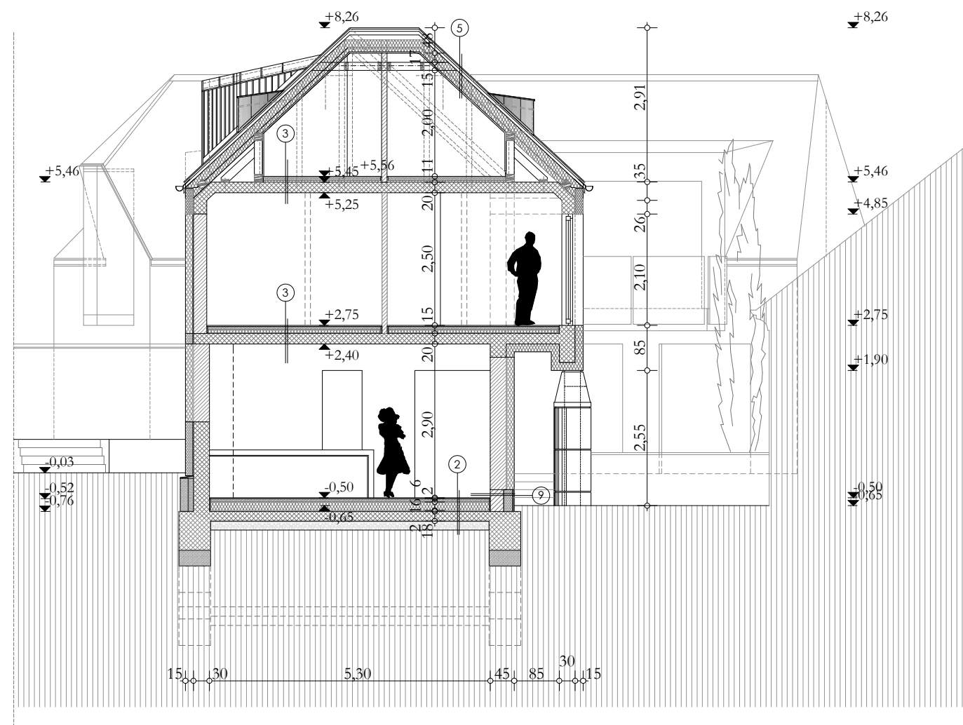
1-1 METSZET
