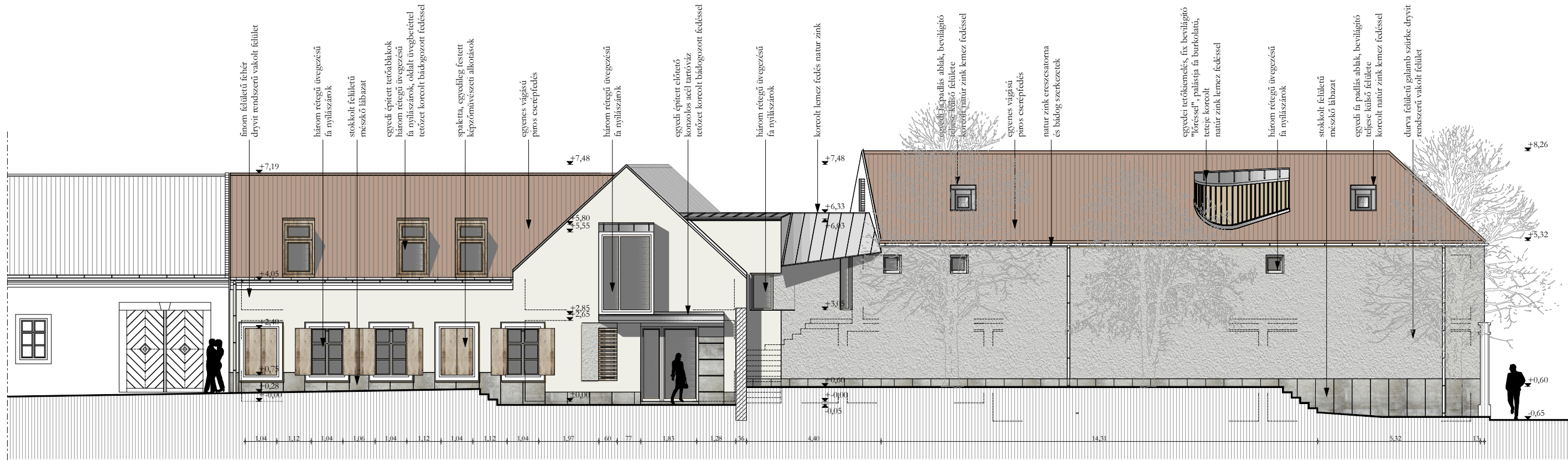
JAKOV IGNATOVITY UTCAI, ÉSZAKI HOMLOKZAT
