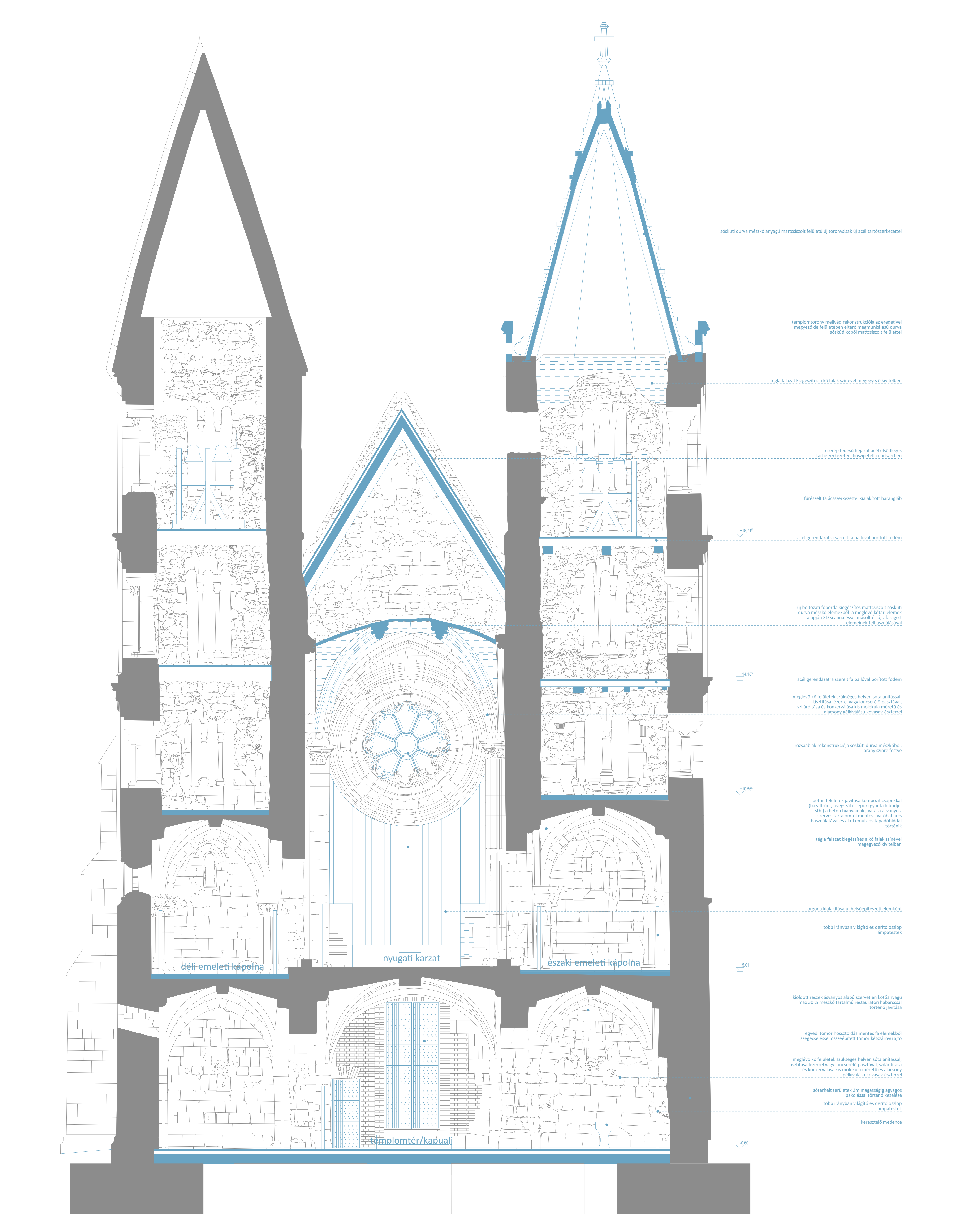
TEMPLOM KERESZTMETSZETE 1:50
