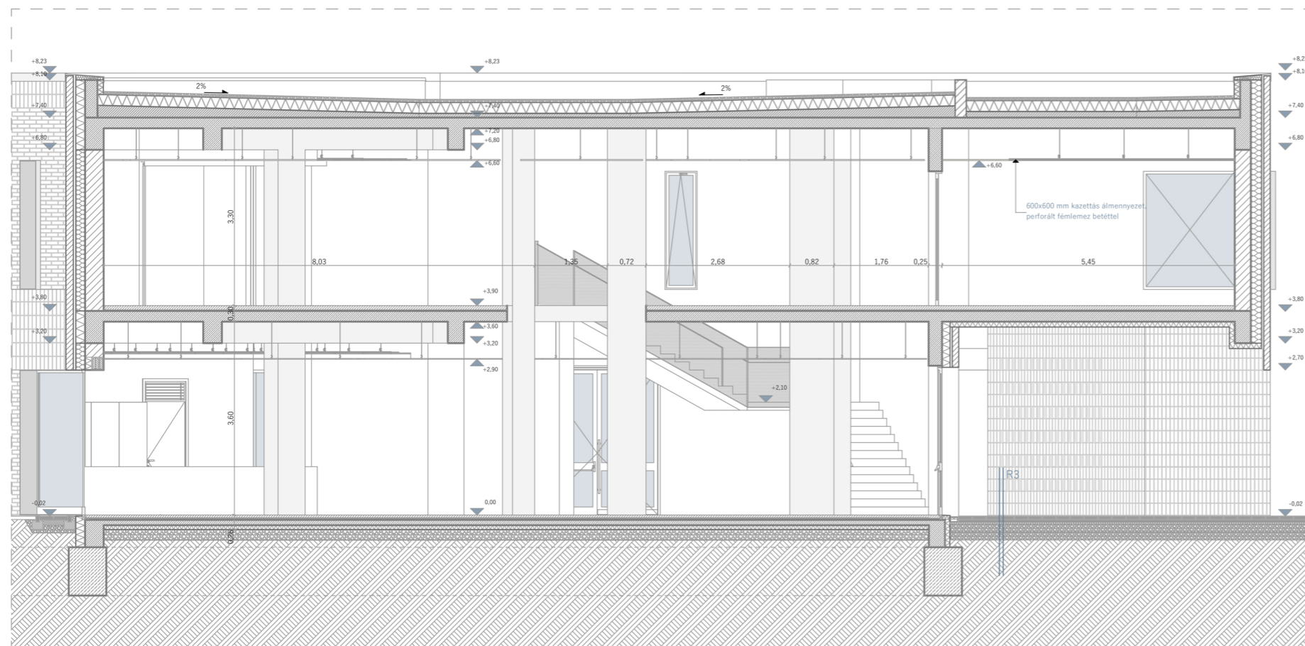
_F-F metszet
