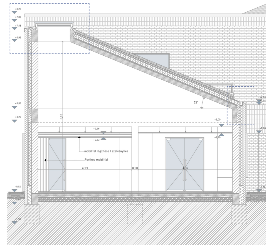
_B-B metszet
