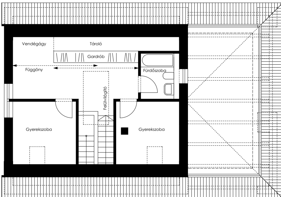
Tetőtéri alaprajz
