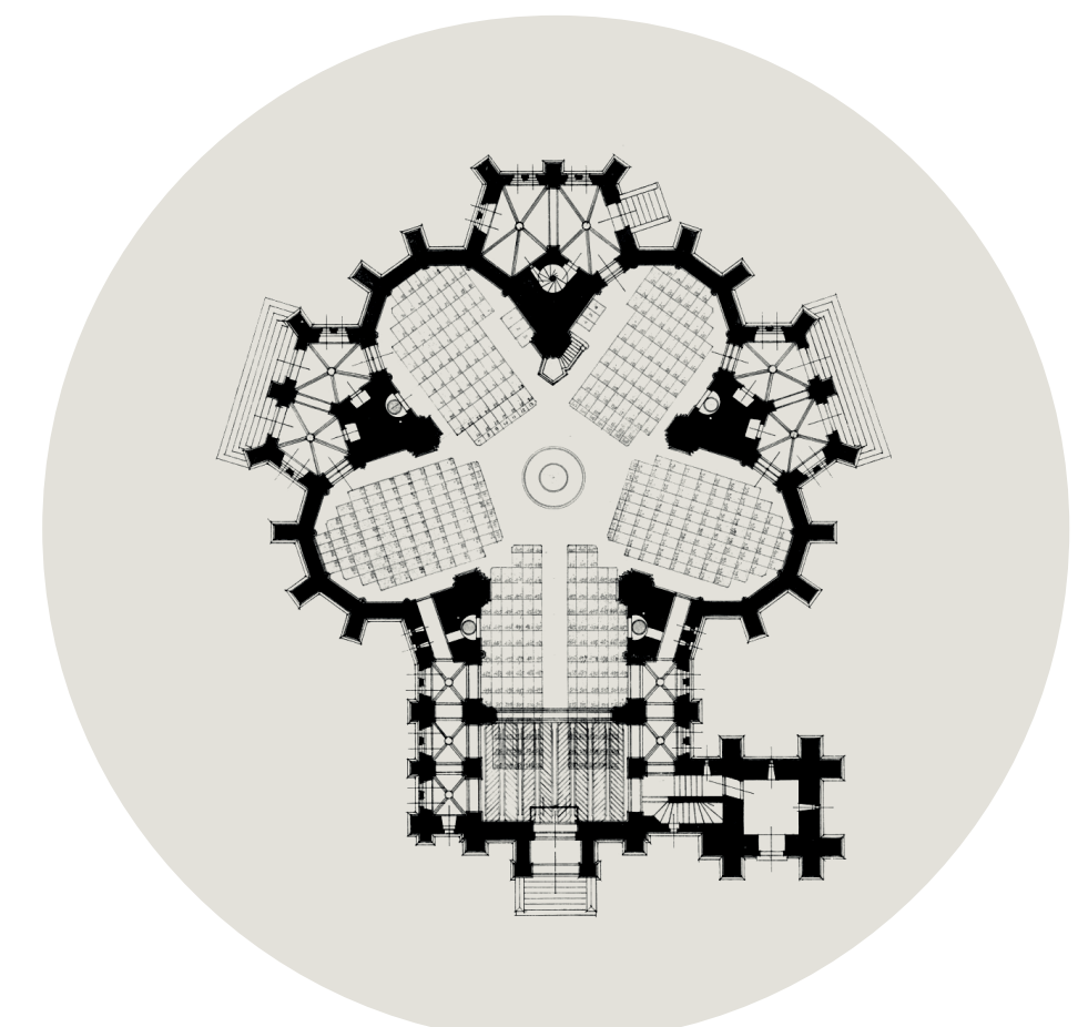
Szilágyi Dezső téri református templom alaprajza (Pecz Samu, 1892)
