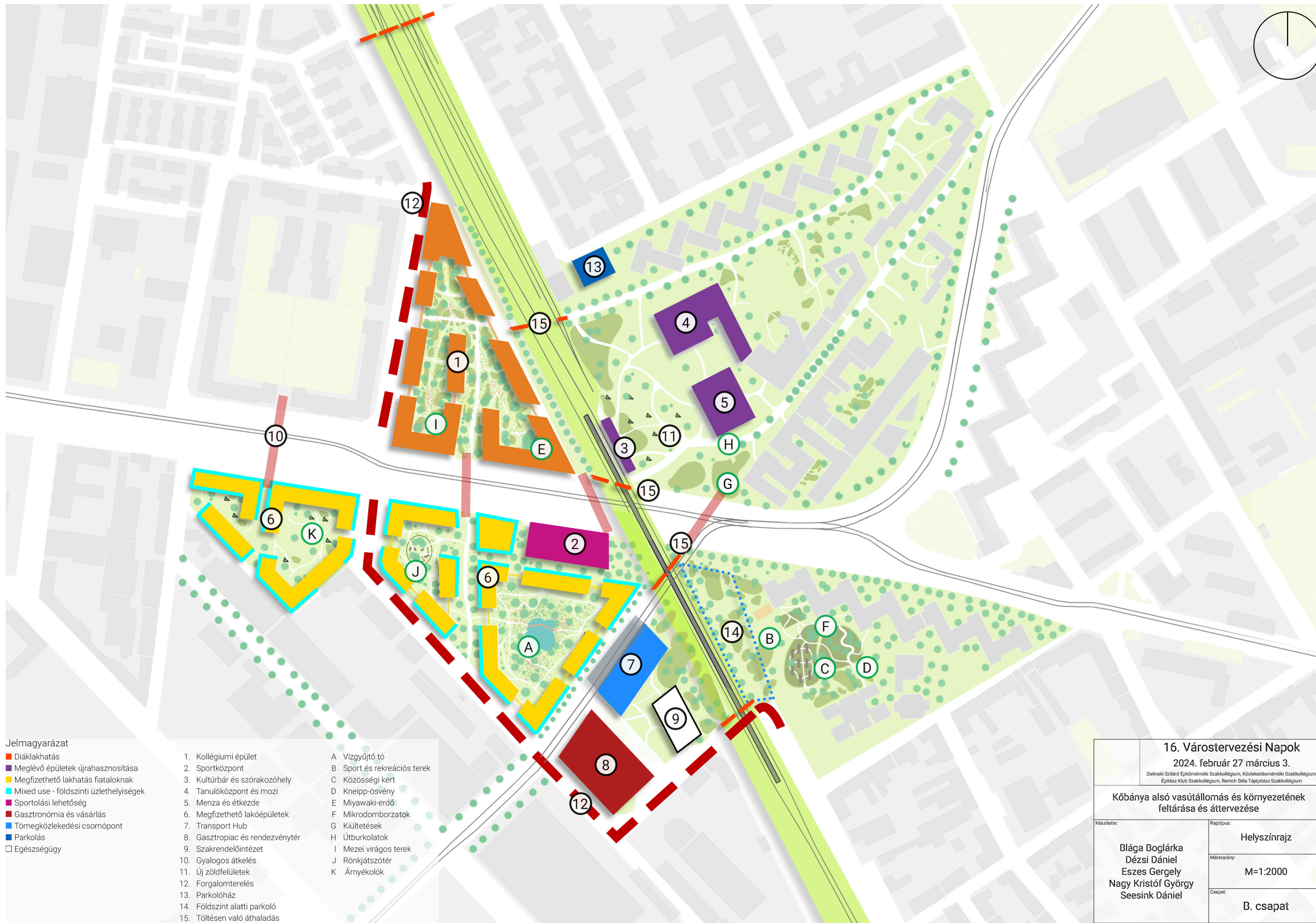
Helyszínrajz
