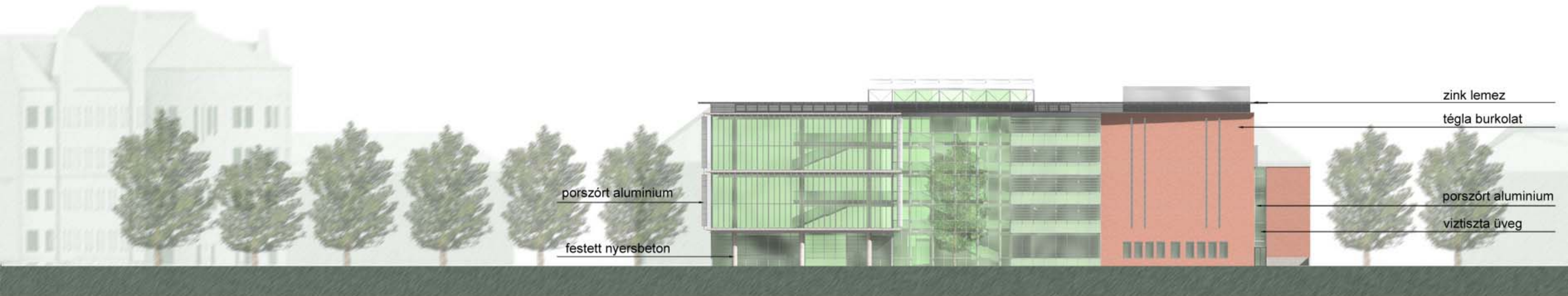
DÉL-NYUGATI HOMLOKZAT
