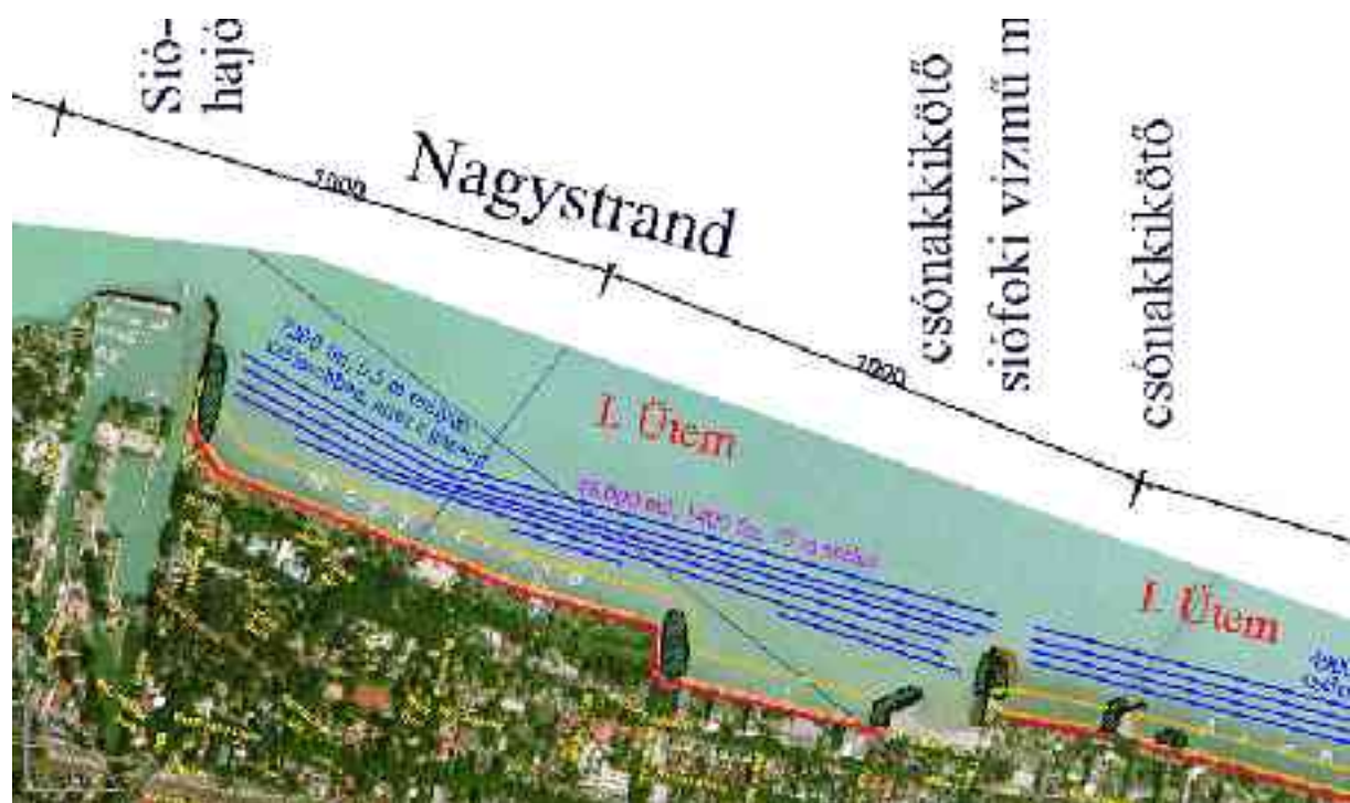
5. A Javaslati tervlap részlete. Sárgával jelölve az új homokpartok határa, pirossal a meglévő betonpartok, késsel a kikotrando homok. (Forrás: A PentaGrid Kft. 1:10000-es méretarányú, 1999-es légifotóra szerkesztett saját rajz)
