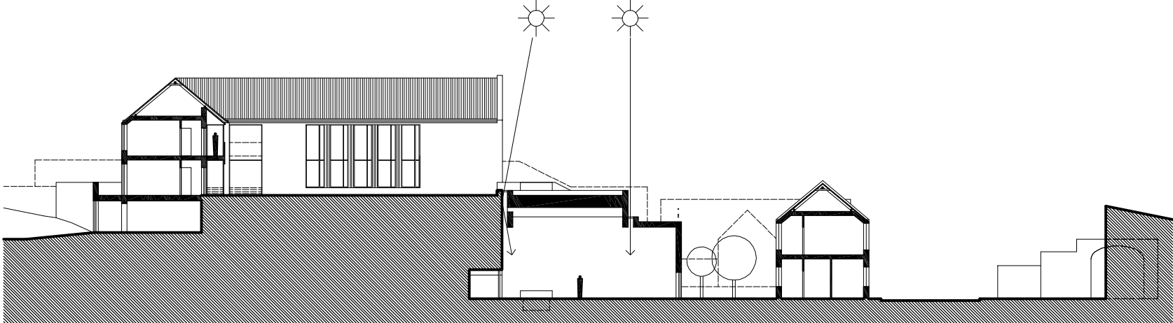
B-B METSZET
