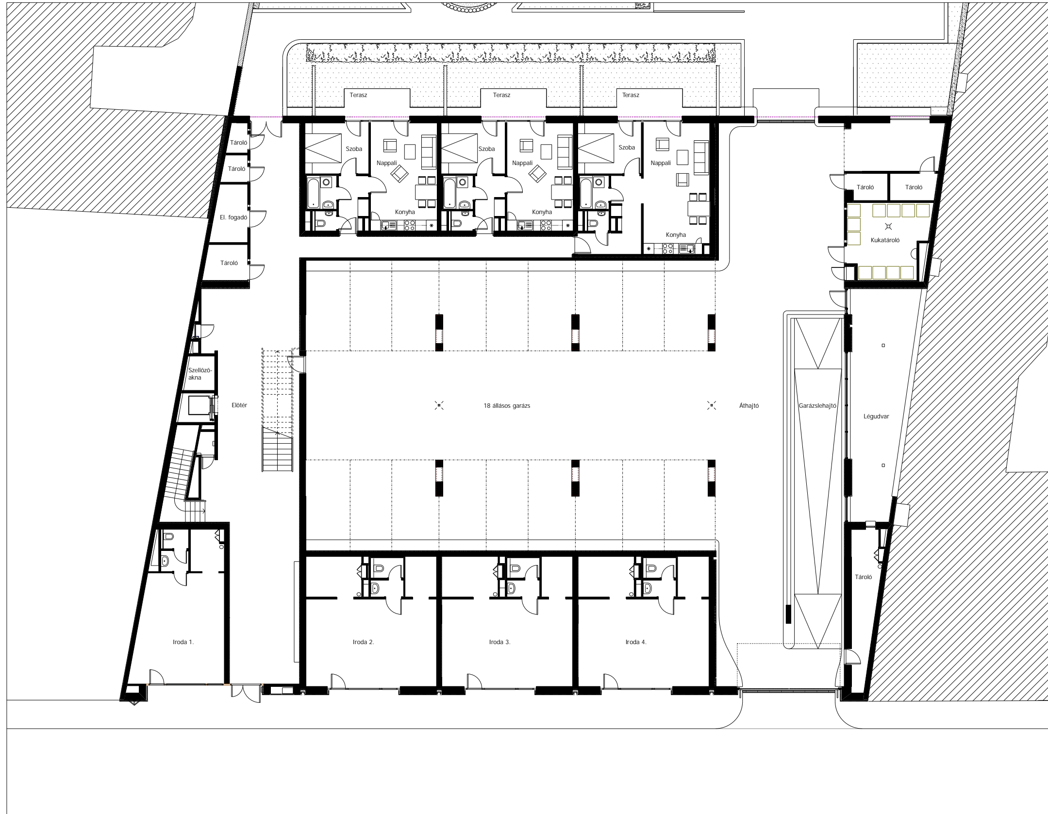
FÖLDSZINTI ALAPRAJZ M1:200
