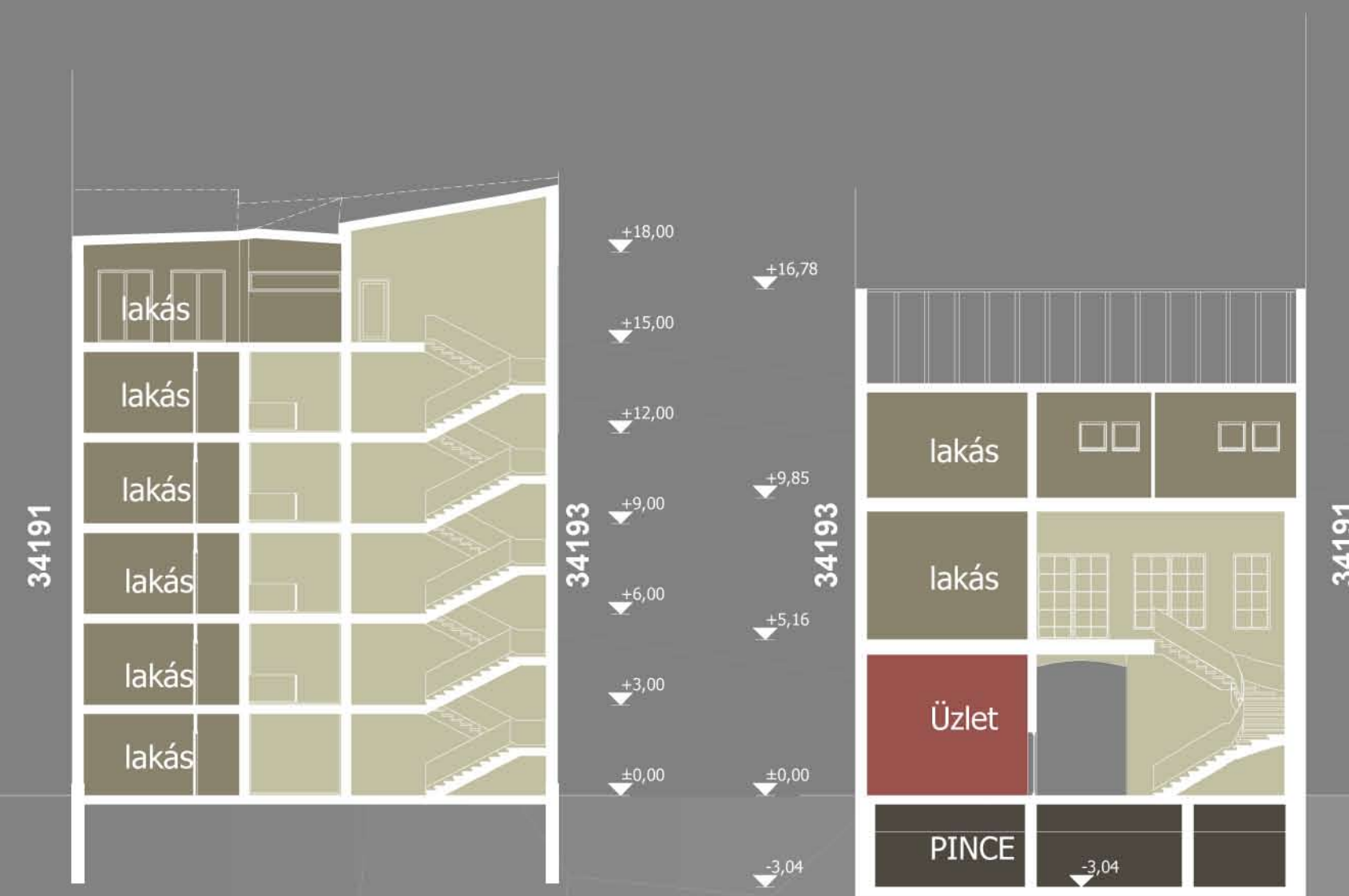
CC metszet BB metszet Dob utca 18 - AA hosszmet szet m 1:200
