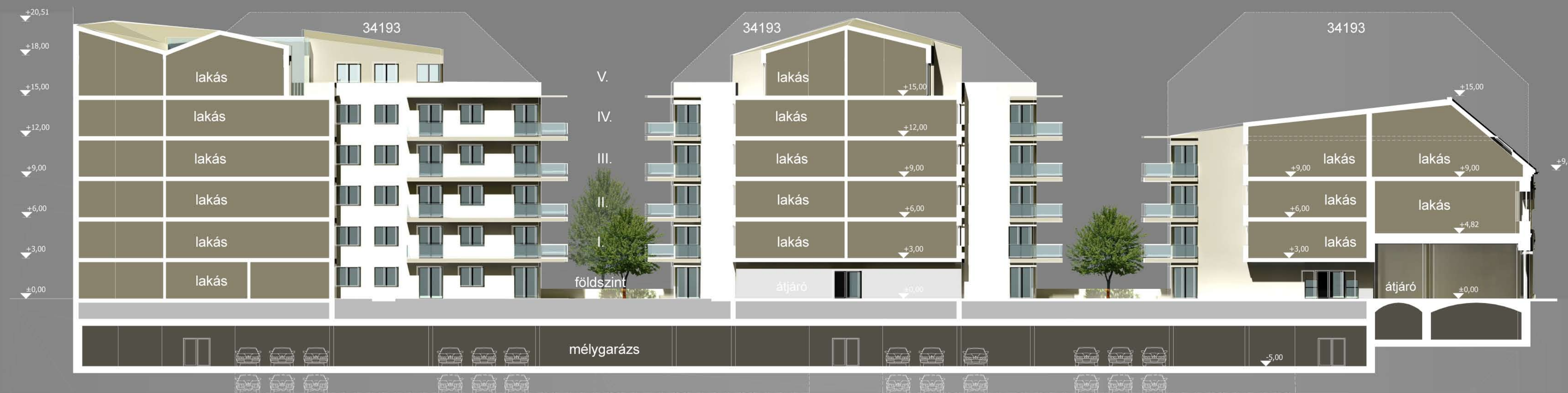
Dob utca 14 - AA hosszmet szet a bels ő udvaron kereszt ü l m 1:200
