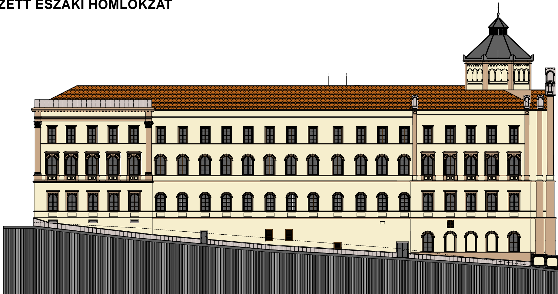
TERVEZETT KELETI HOMLOKZAT
