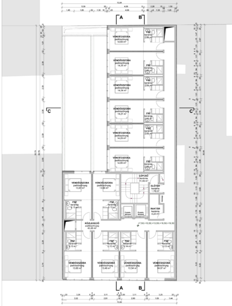
ÁLTALÁNOS EMELETI ALAPRAJZ, M1:100
