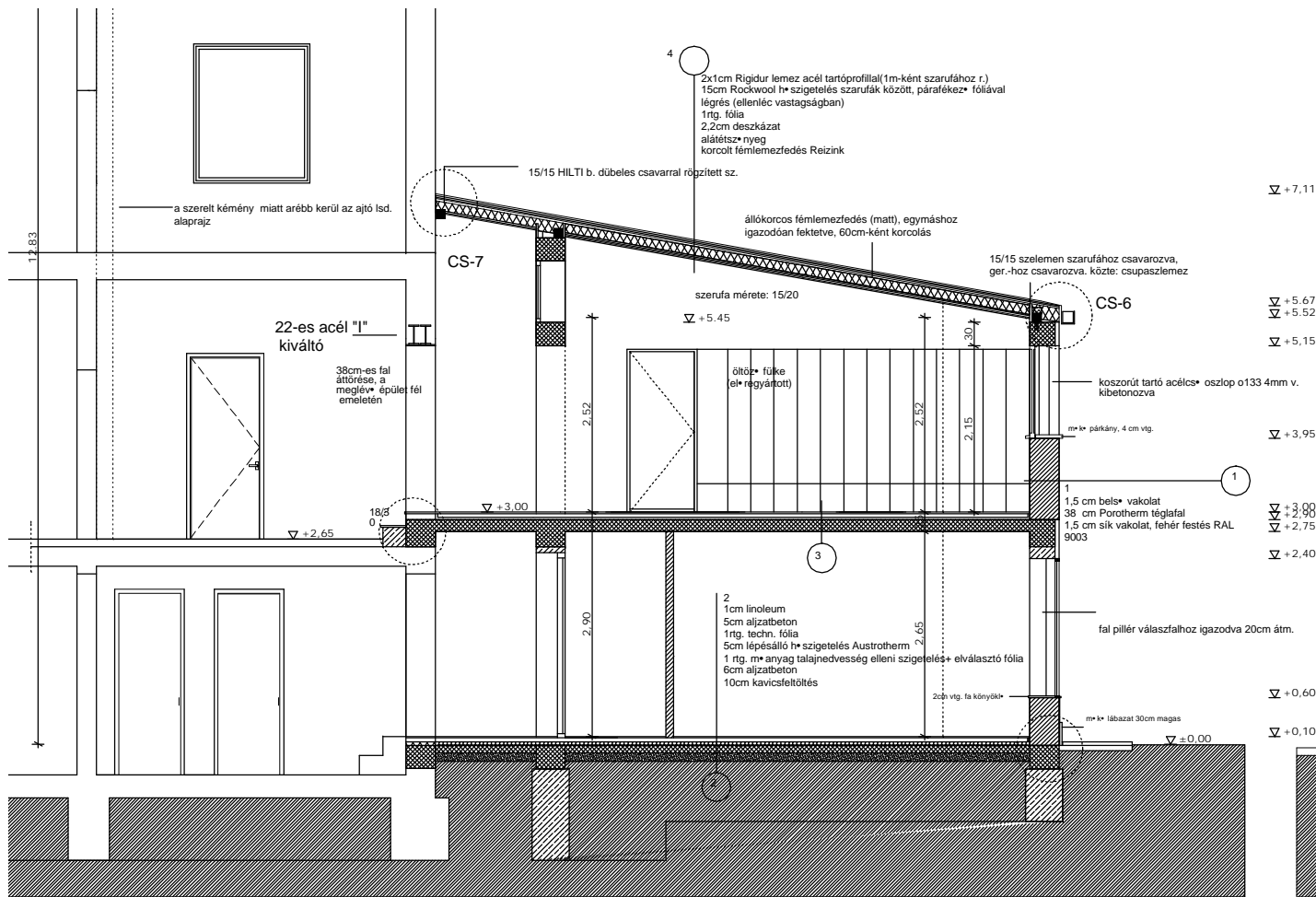
B-B metszet M1 1:100
