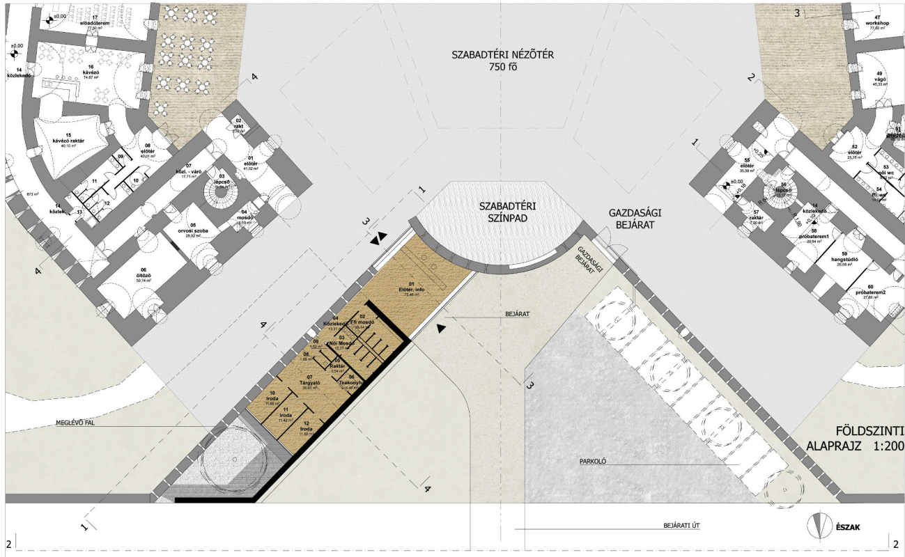
FÖLDSZINTI ALAPRAJZ 1:200
