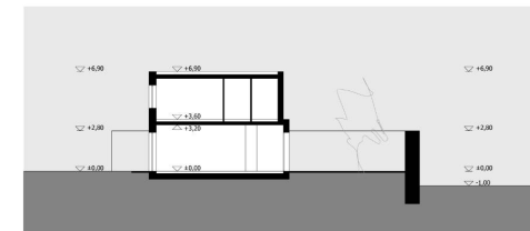
4-4 METSZET 1:200
