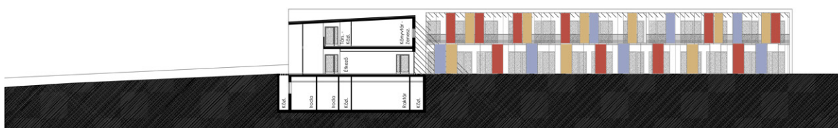
délkeleti (udvari) homlokzat és metszet m 1:200
