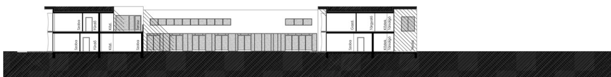
északkeleti (udvari) homlokzat és metszet m 1:200
