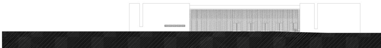
délnyugati (Alacscai úti) homlokzat m 1:200
