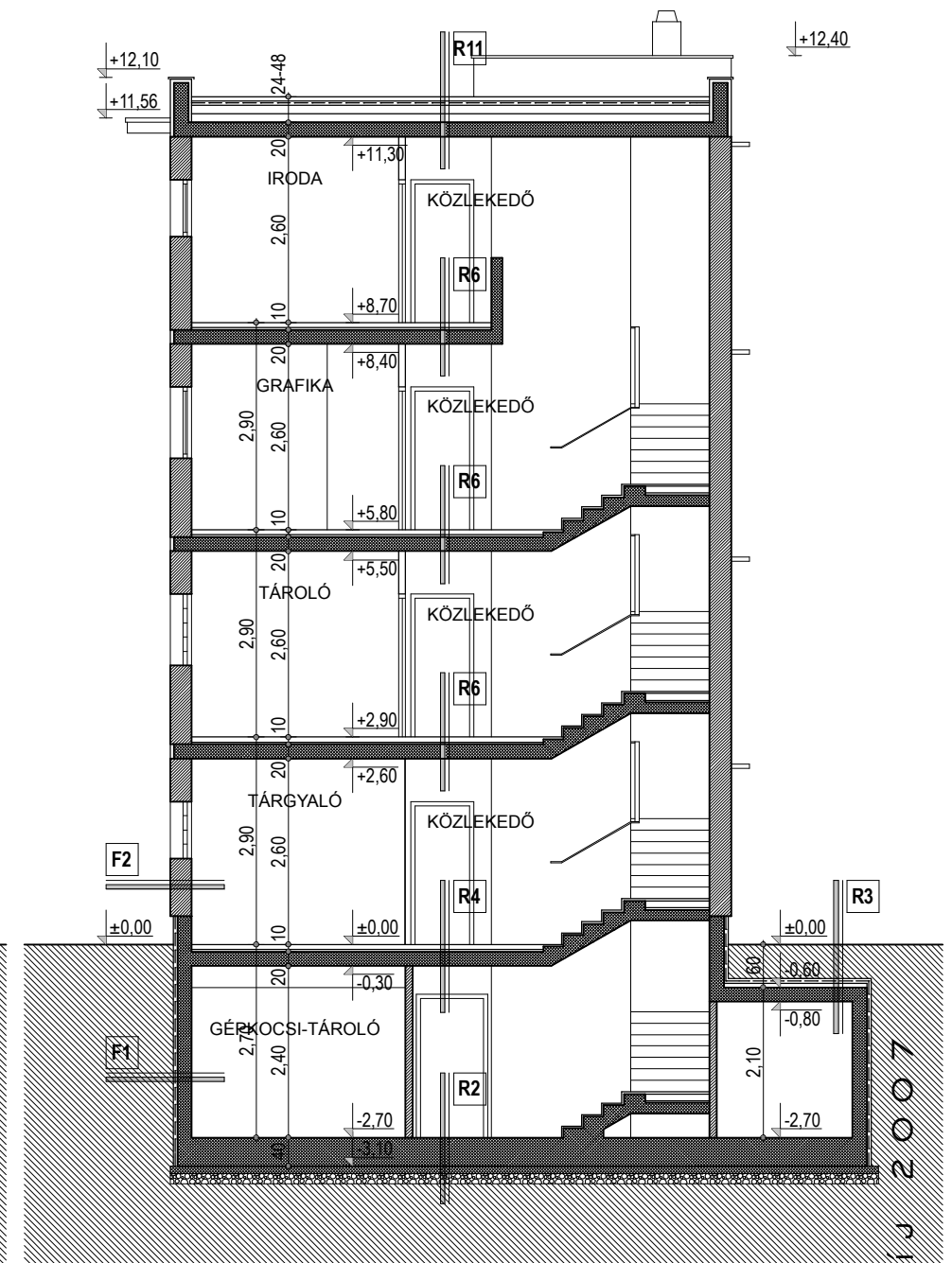
B-B METSZET
