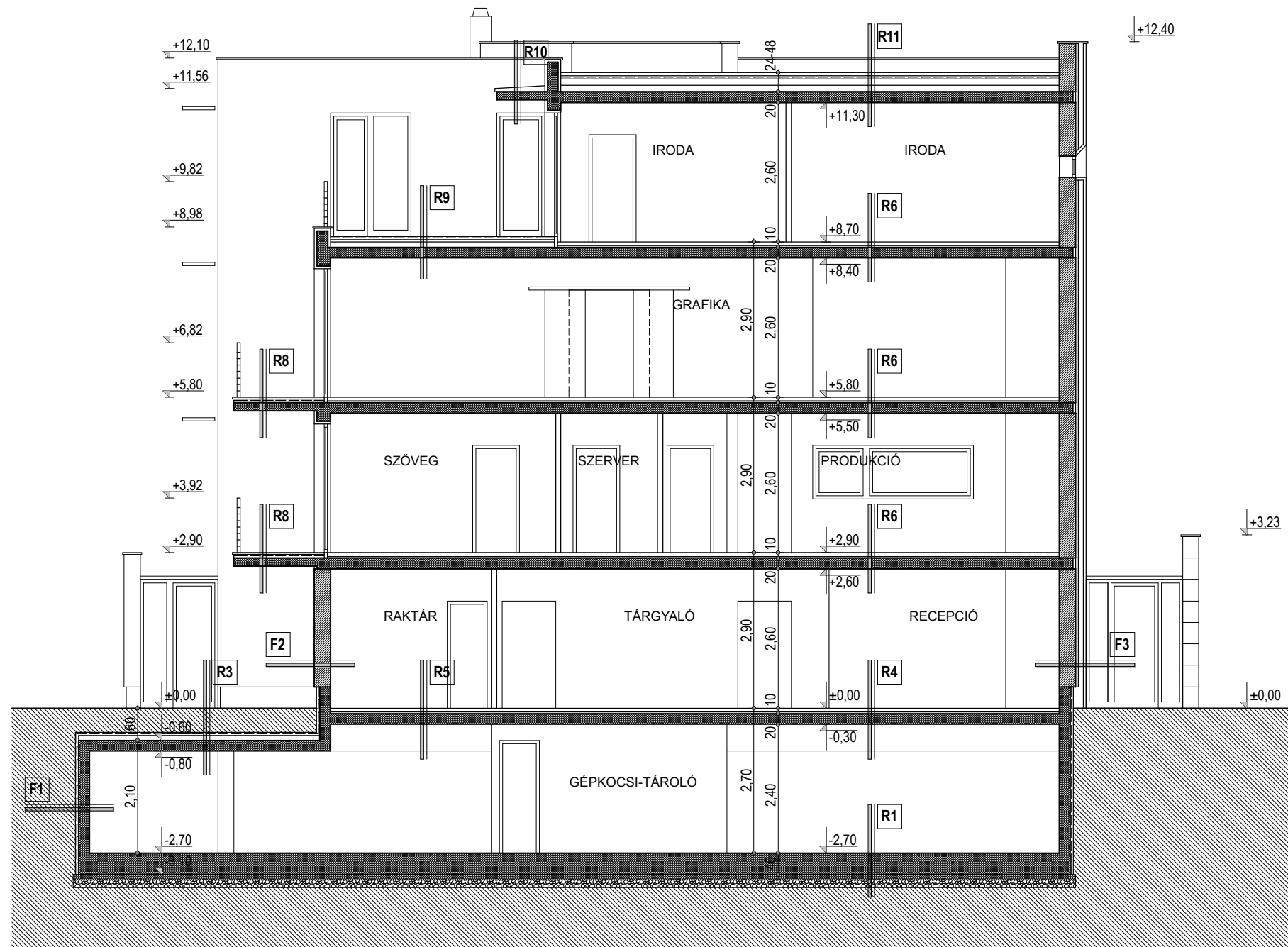
A-A METSZET
