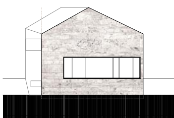
nyugati homlokzat
