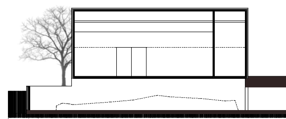
hosszmetszet
