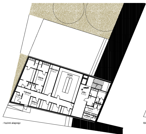
panzió alaprajzai, metszet, homlokzatok m1_200
