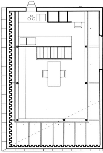
二階平面図 2F PLAN
