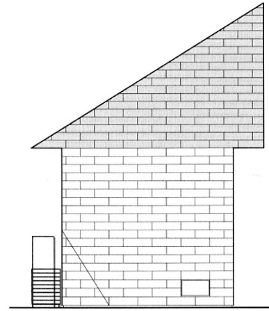
立面図 ELEVATION
