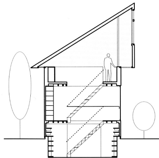
断面図 SECTION
