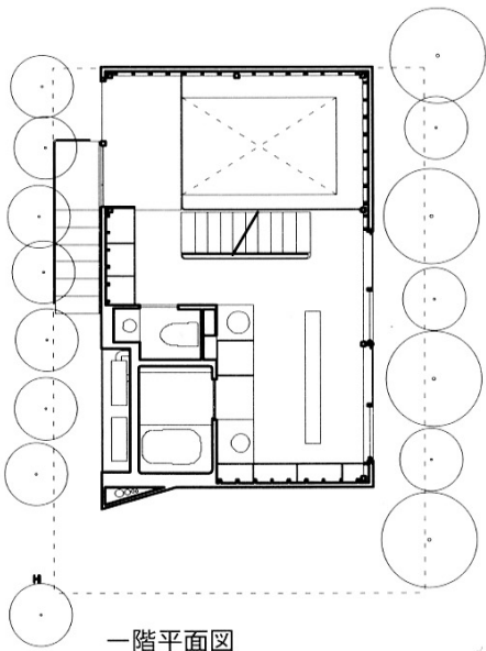
一階平面図 1F PLAN
