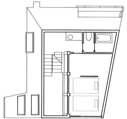
三階平面図 3F PLAN
