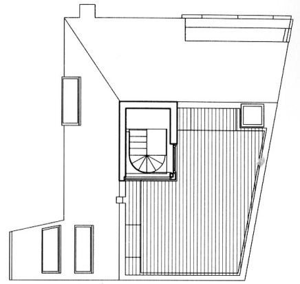
屋上平面図 RF PLAN
