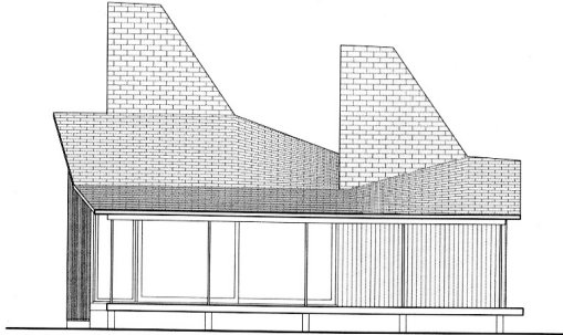
立面图 ELEVATION
