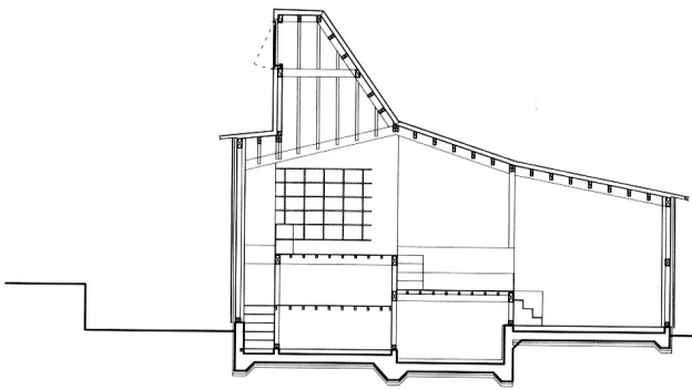
断面图 SECTION
