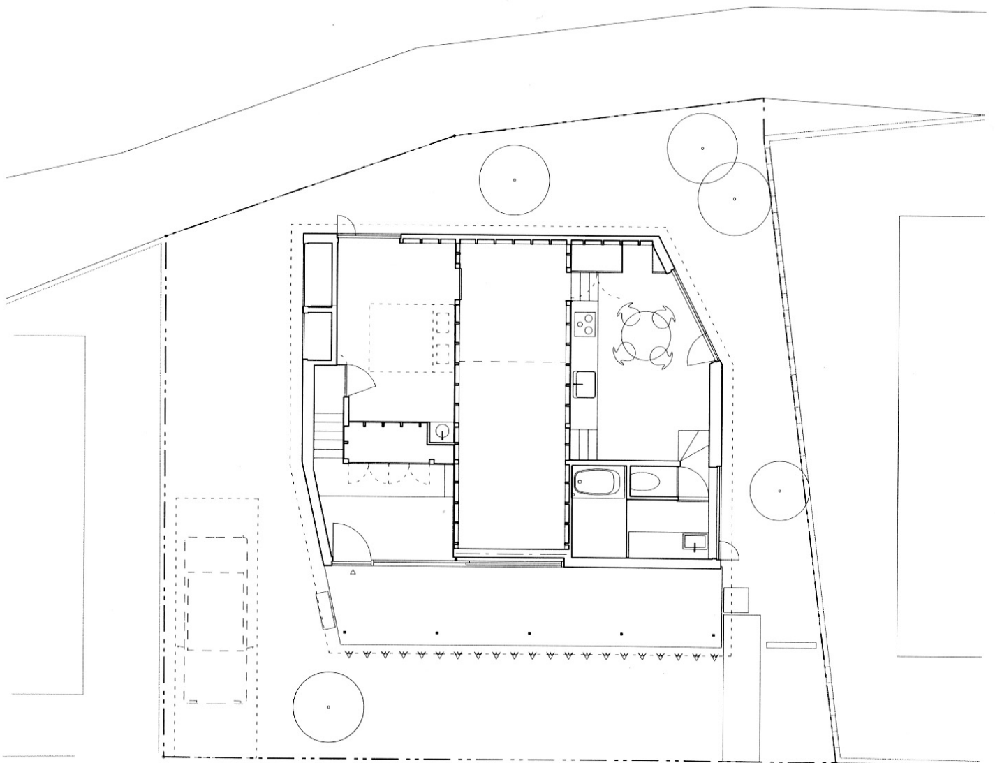
下部平面図 LOWER PART PLAN
