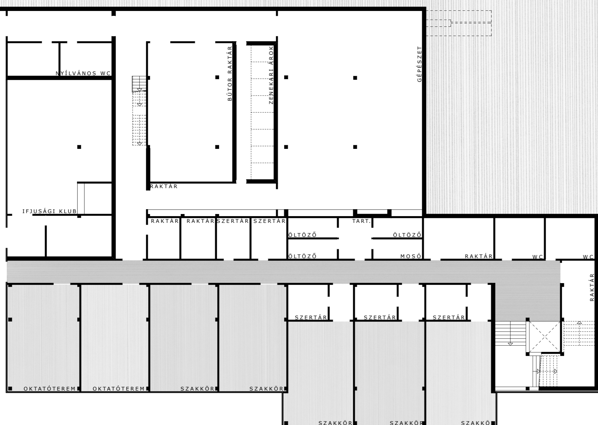
FÖLDSZINTI ALAPRAJZ
