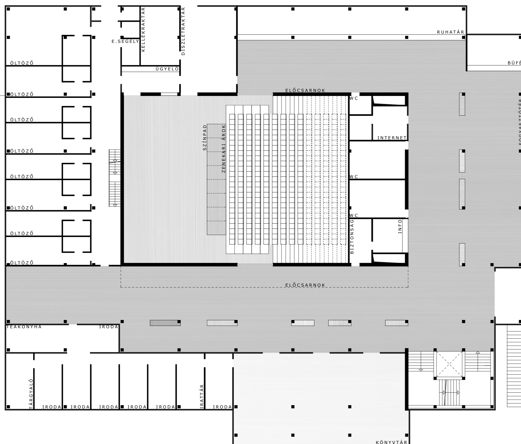
I.EMELETI ALAPRAJZ
