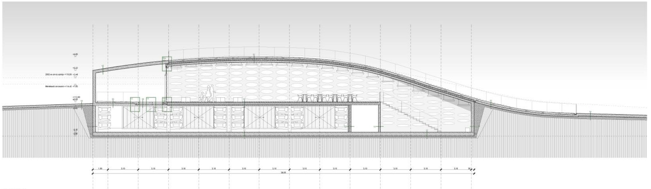
B metszet
