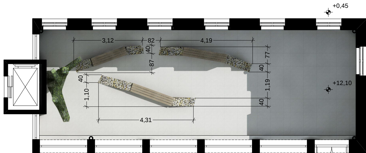
ALAPRAJZ M 1:100
