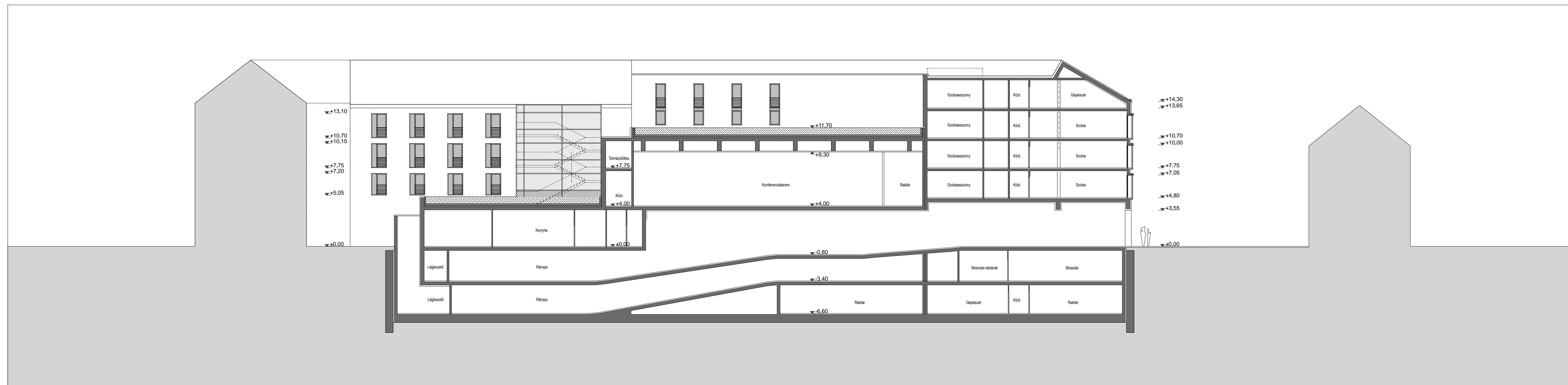
A-A METSZET
