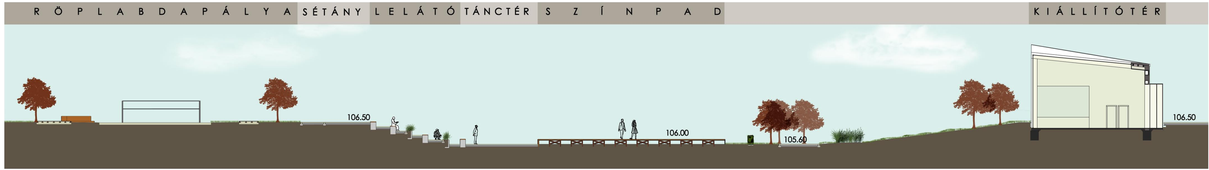
C - C METSZET 1.
