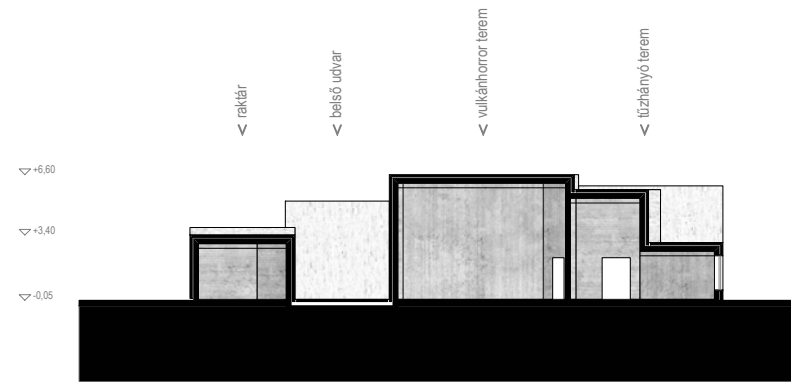
3_3 metszet m 1_200
