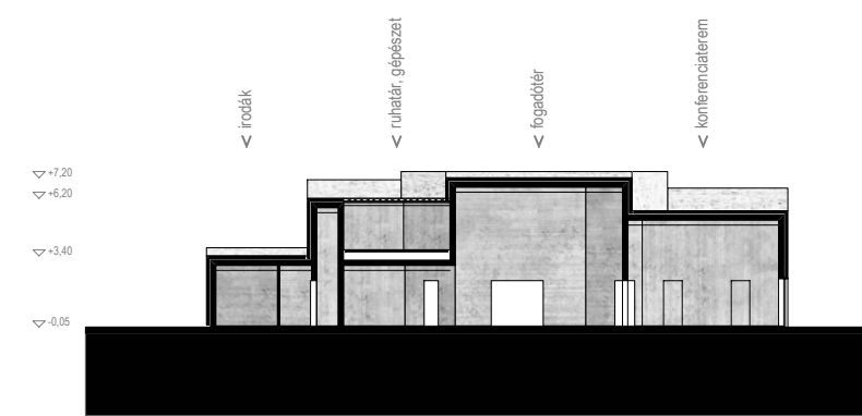
5_5 metszet m 1_200
