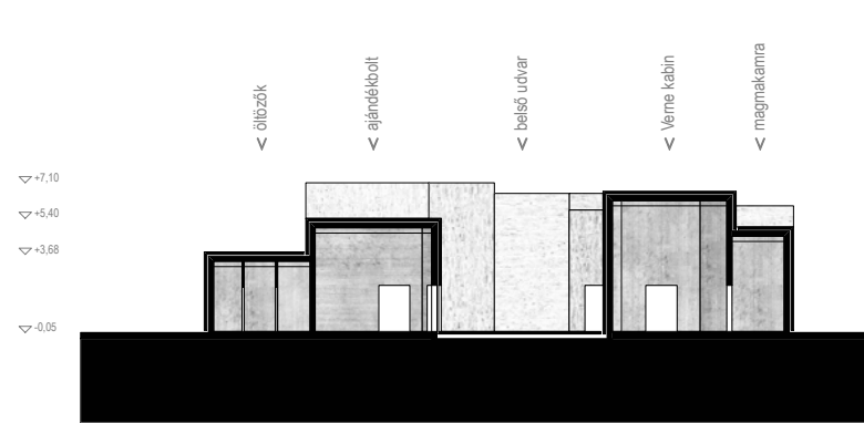
4_4 metszet m 1_200
