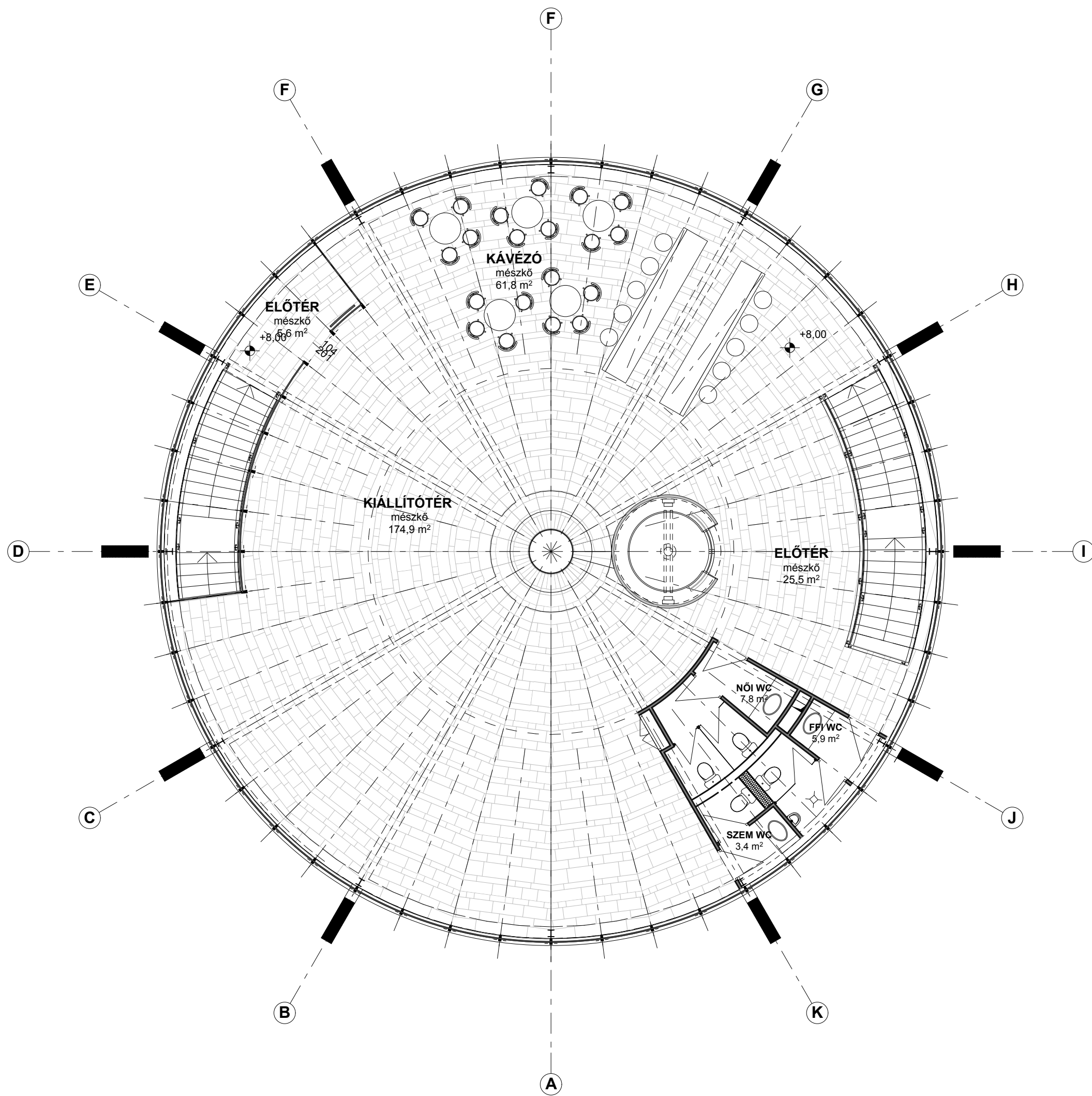
+8,00 SZINT ALAPRAJZA 1 : 100
