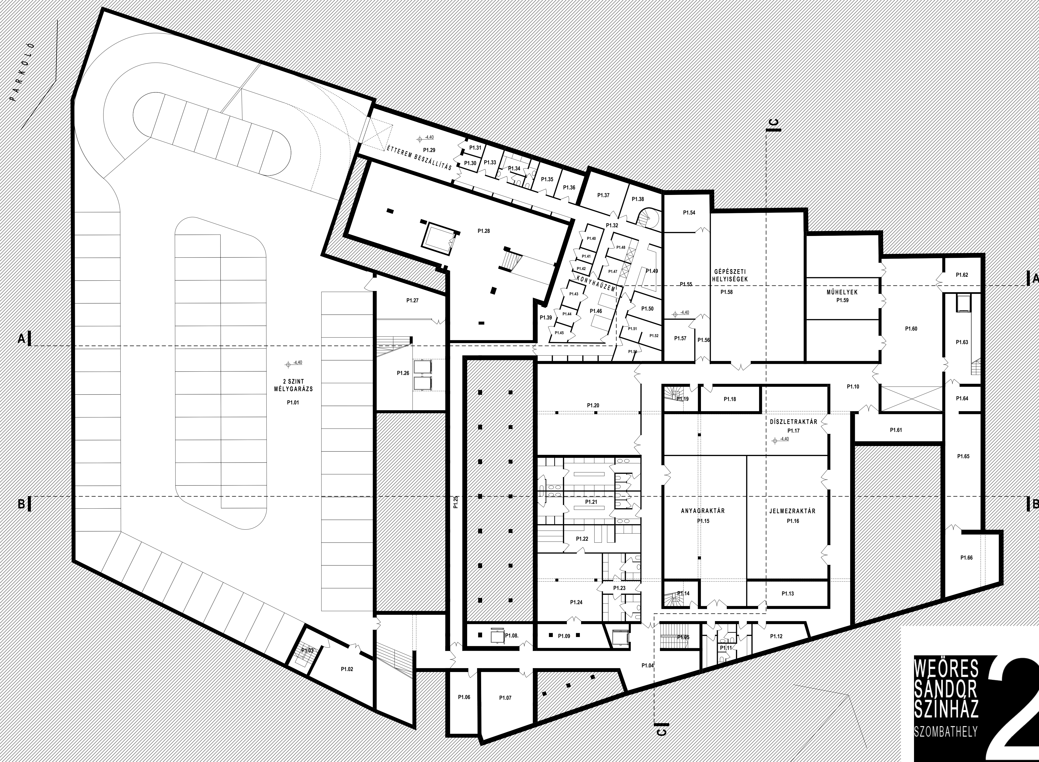
PINCESZINTI ALAPRAJZ M 1:200
