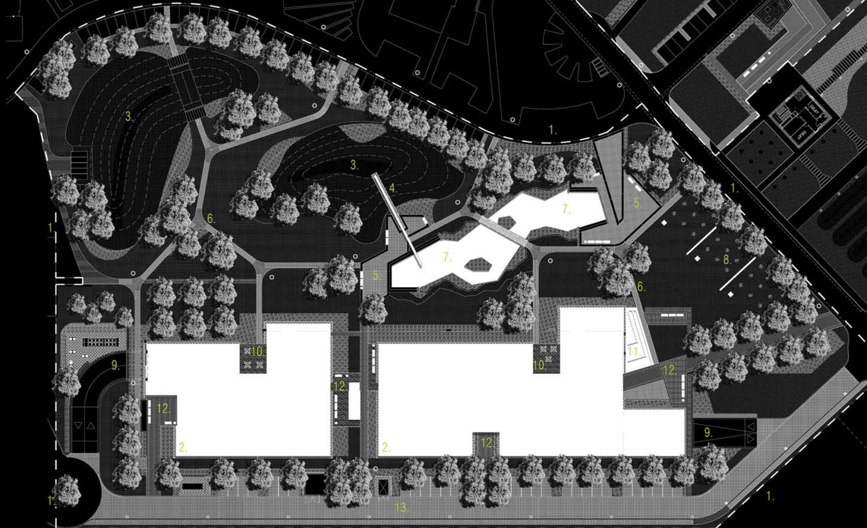
M=1:500 1. tervhatar, 2. 'M'-epulet, 3. mesterséges domb (tervezési adottság), 4. vízesésfal, 5. tér, 6. gyalogos úthálózat, 7. tó, 8. buxusraszter, 9. mélygarázs lejárata, 10. faburkolatú terasz, 11. kaszkád medence, 12. gyalogos bejárata, 13. kiszolgáló út
