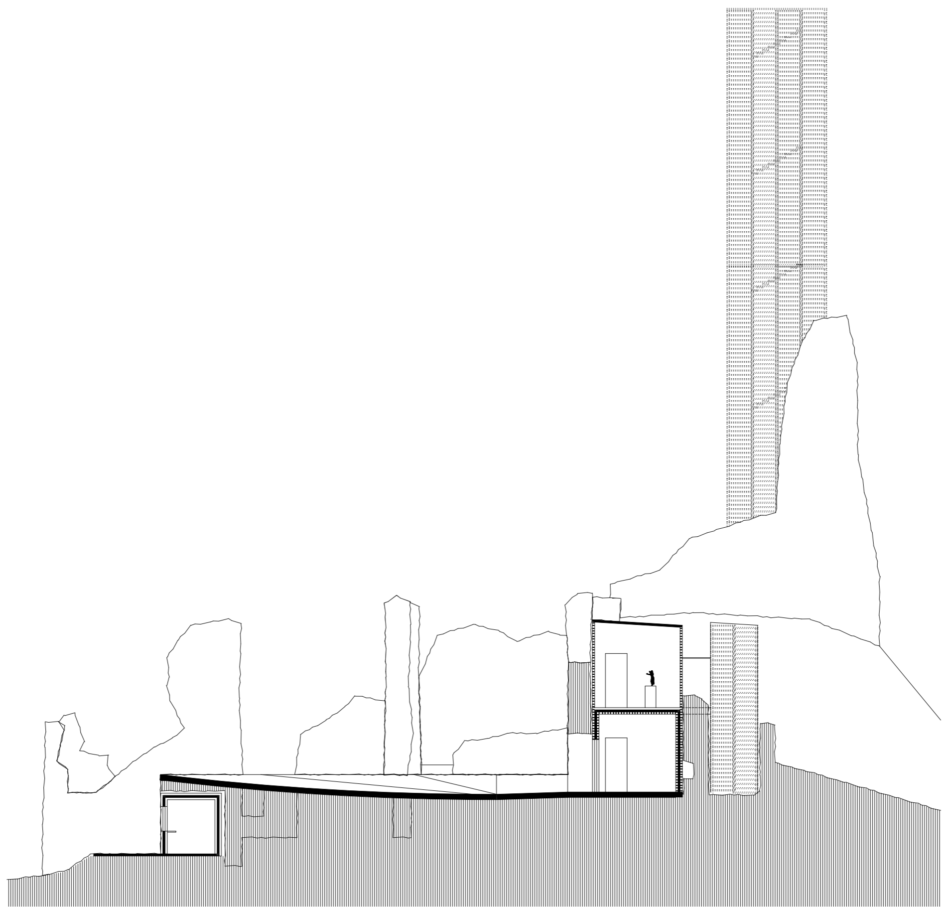
BB metszet m 1:200
