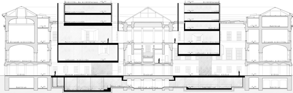
A A METSZET M1:250
