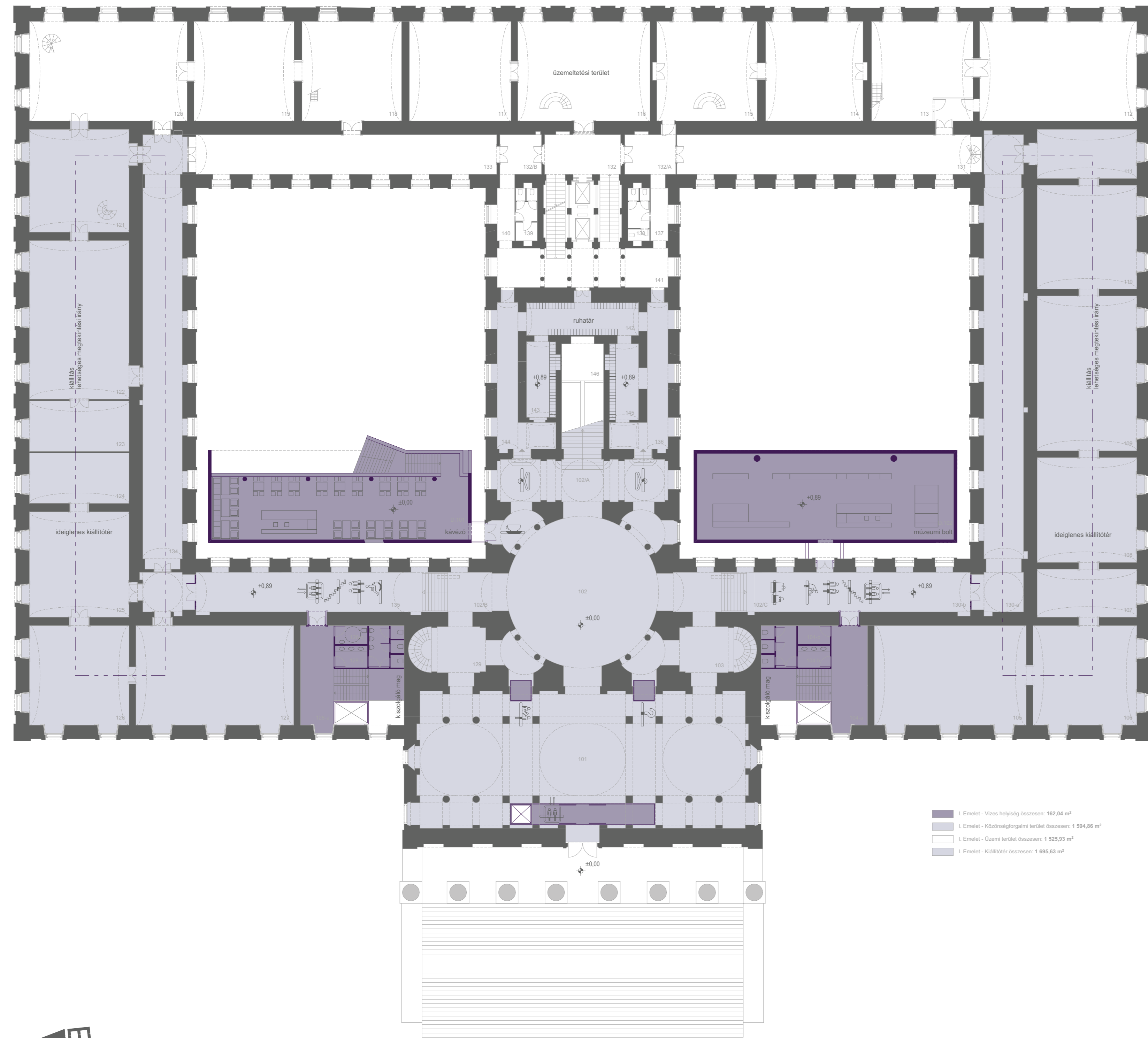
_első szint alaprajz_ 1:250
