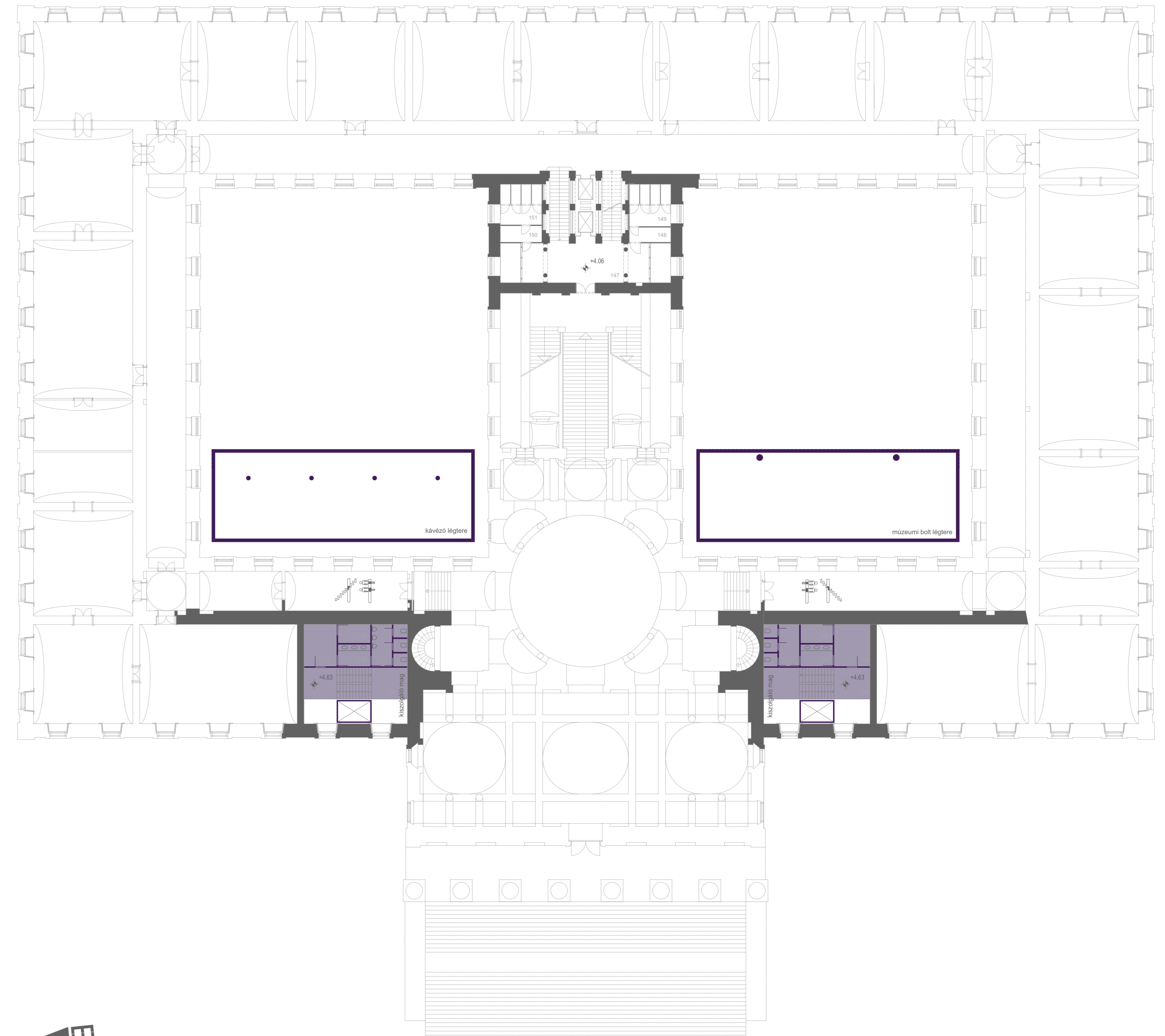
_első emelet feletti félszint alaprajz_ 1:250
