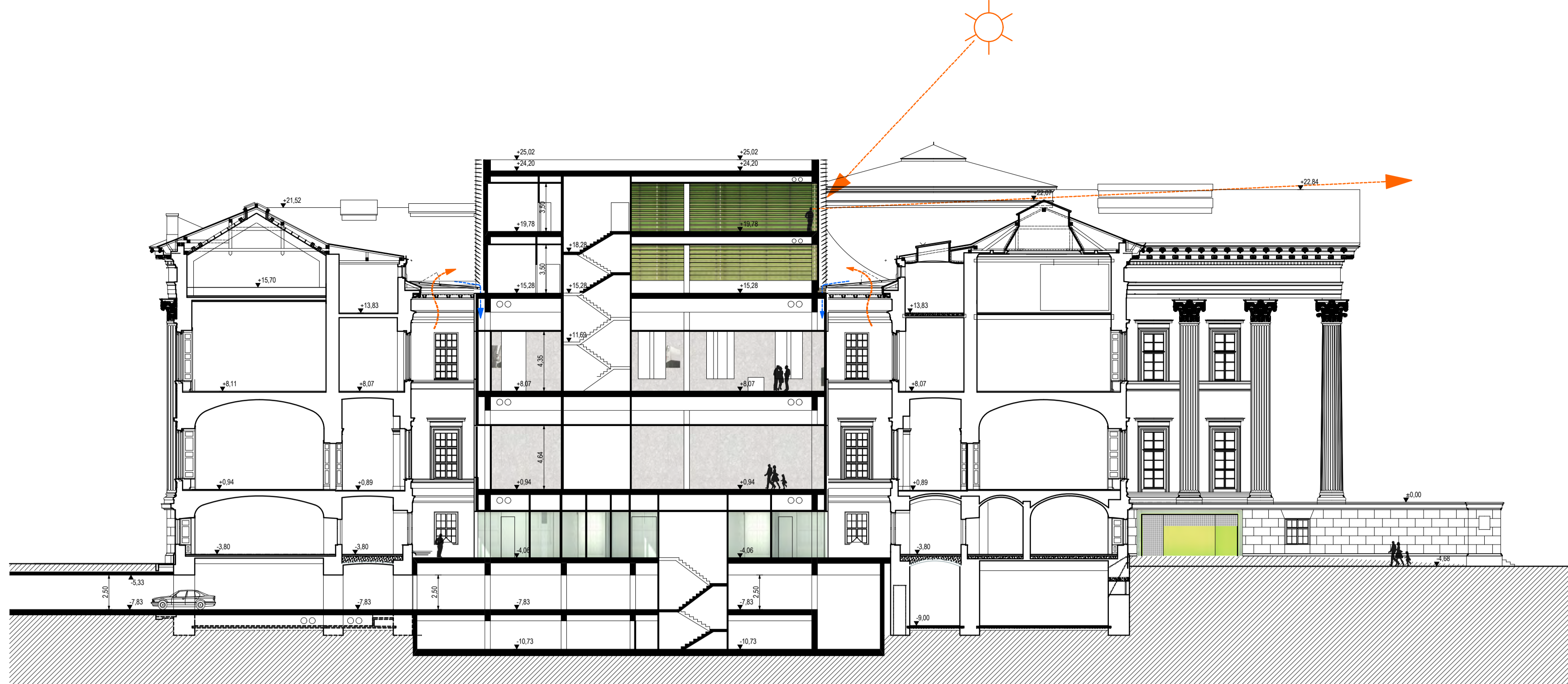
2-2 METSZET
