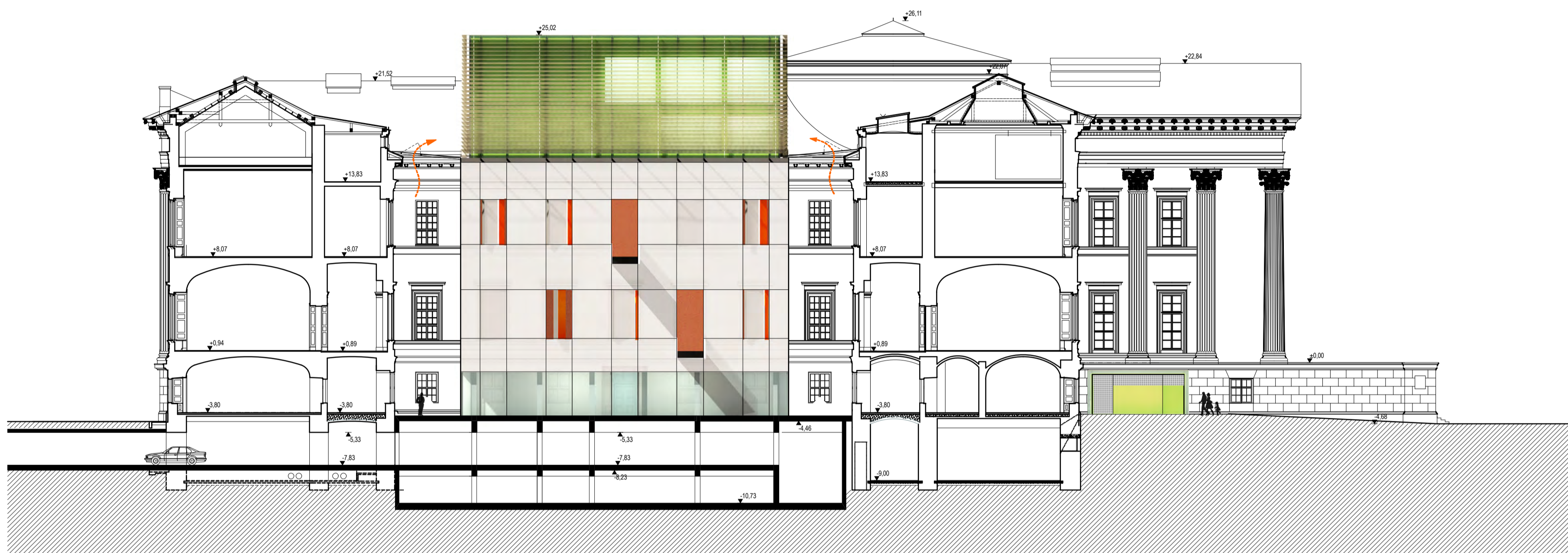
UDVARI HOMLOKZAT - BŐVÍTÉNY
